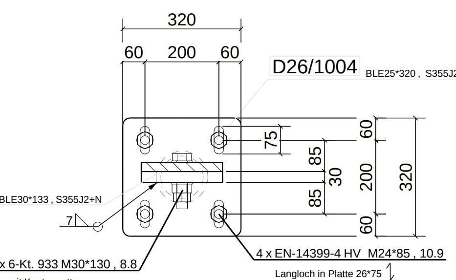
DETAIL 5, Schnitt H - H 3: bergseitiger Stützenfuss (S2/S3)
