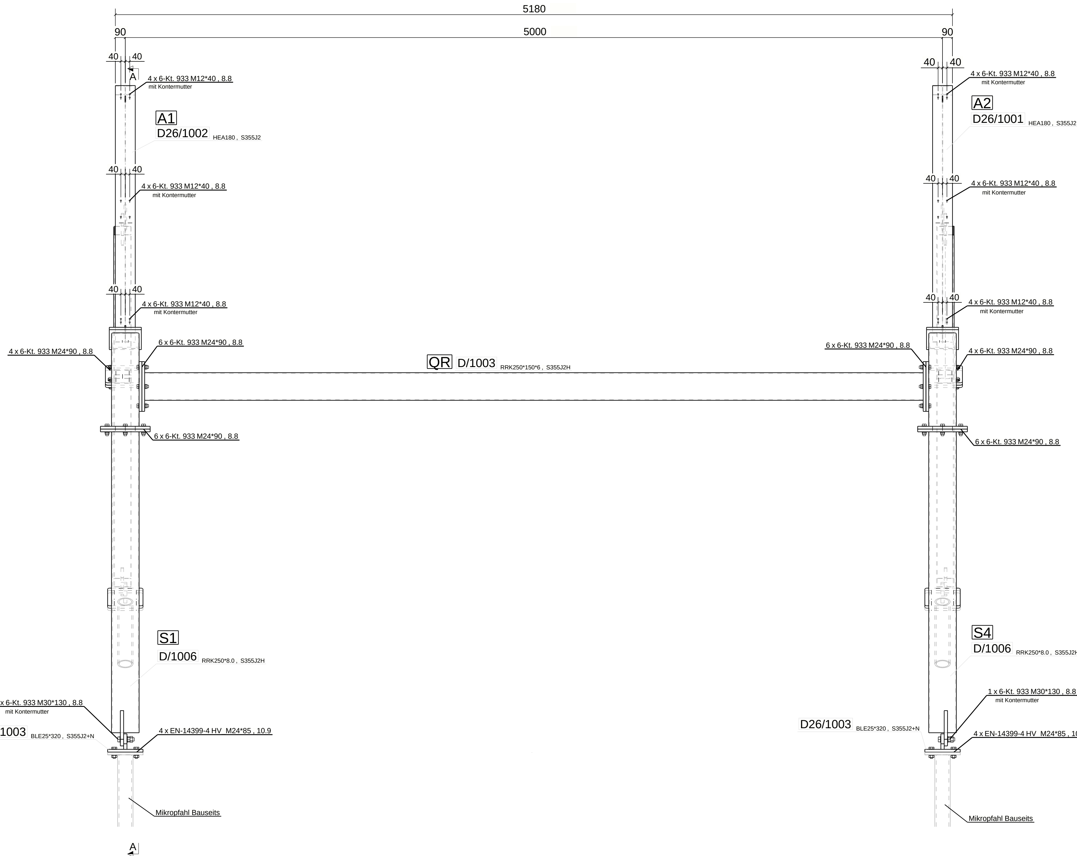
Ansicht: Primärkonstruktion Typ D - 2026 1:20
