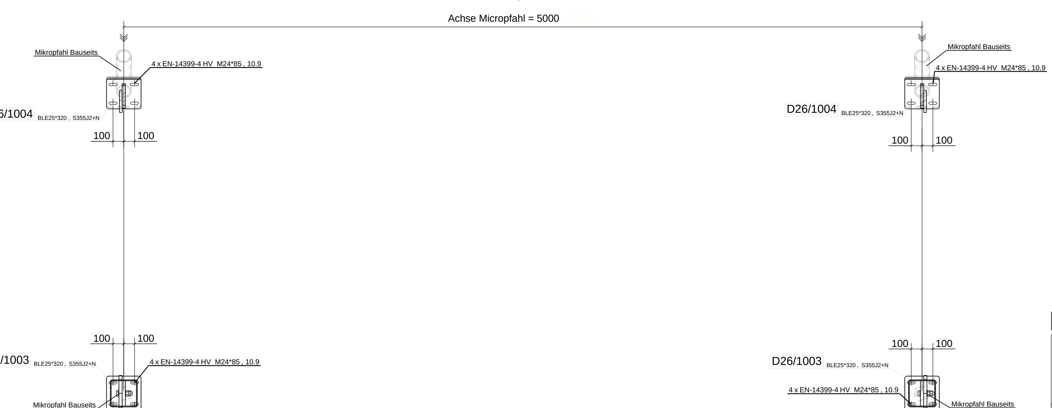
Grundriss: Primärkonstruktion Typ D - 2026 1:20
