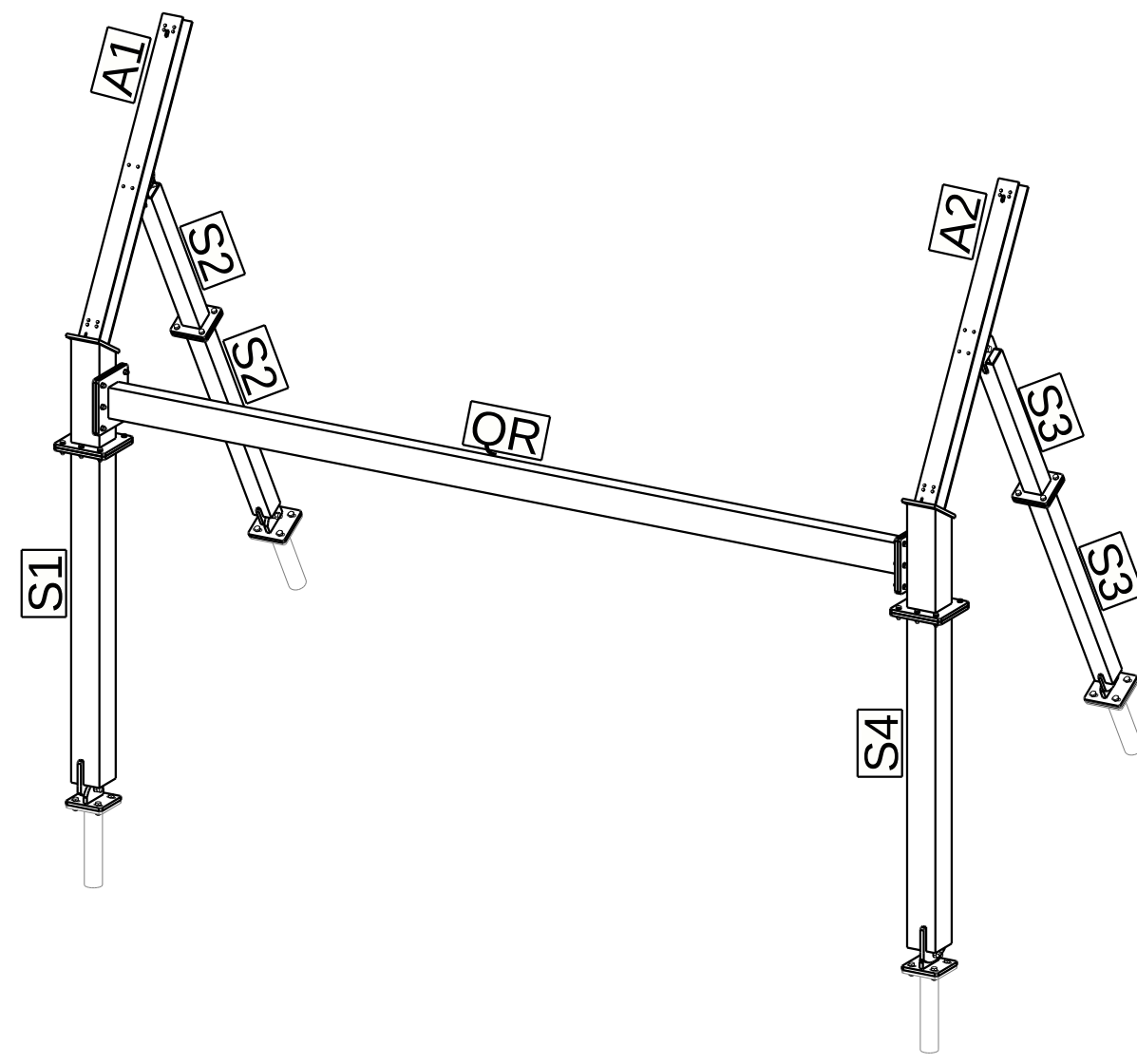
Isometrie Primärkonstruktion Typ D - 2026 1:55
