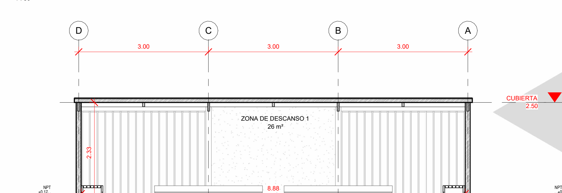
8 CORTE C 1 : 50
