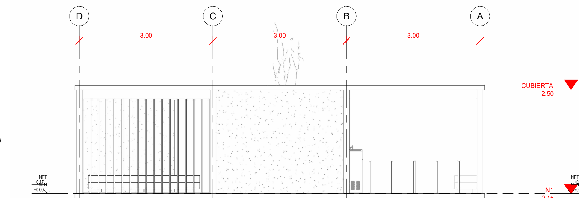
4 ELEVACIÓN 3 1 : 50
