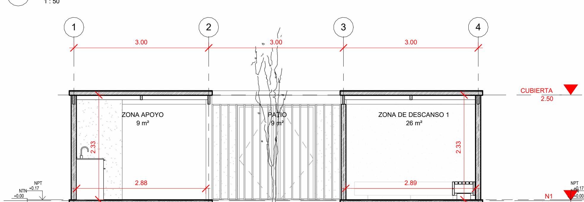
9 CORTE B 1 : 50
