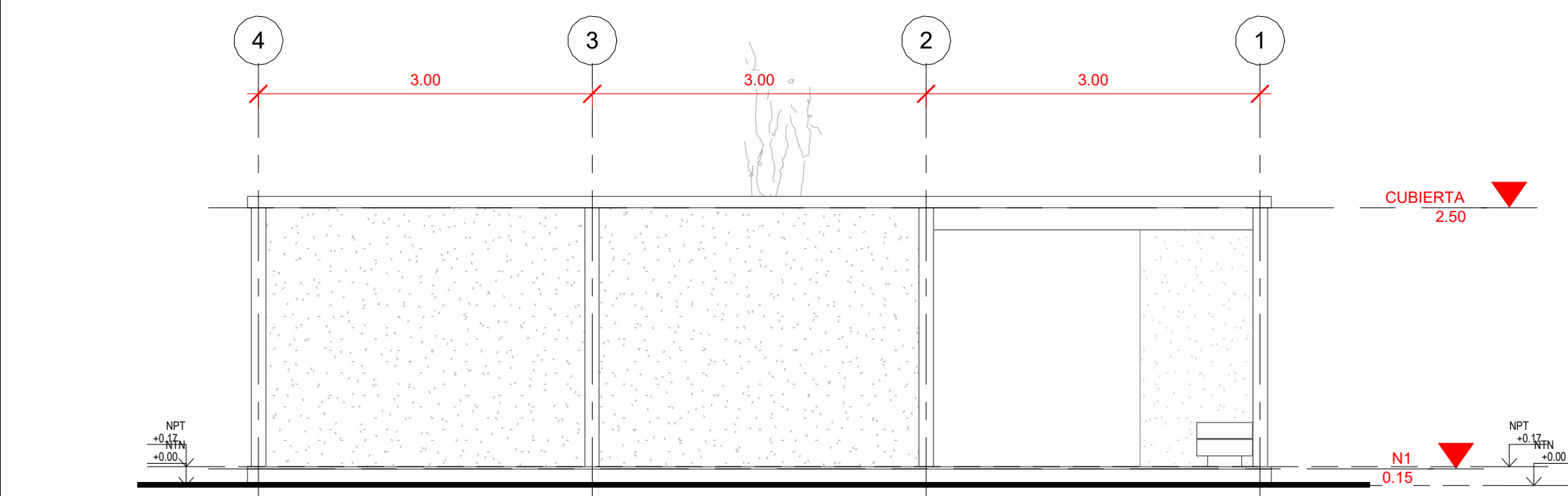
3 ELEVACIÓN 2 1 : 50
