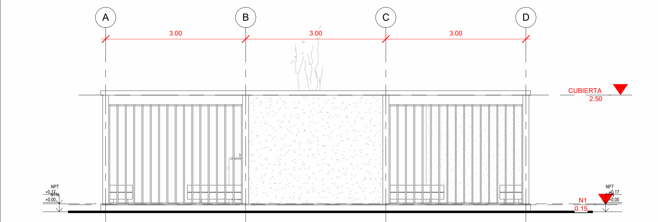
2 ELEVACIÓN 1 1 : 50
