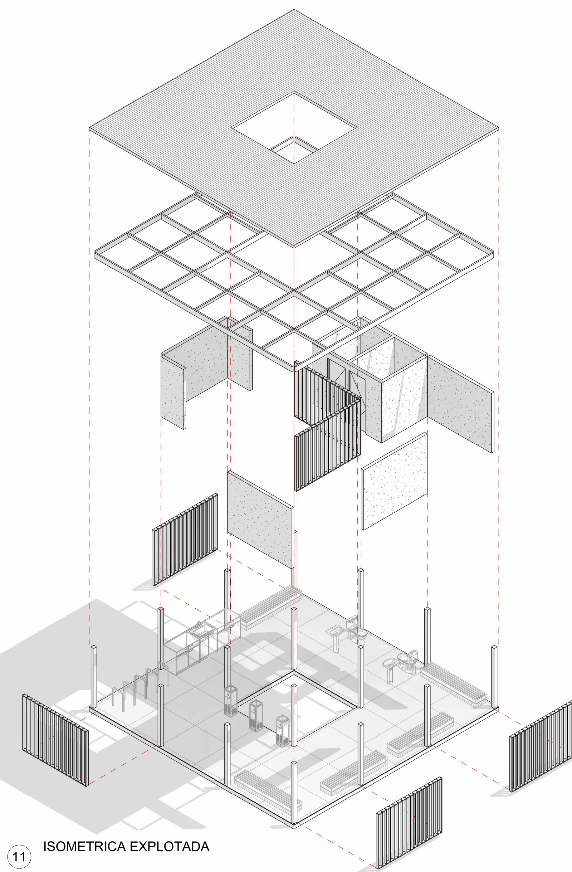
11 ISOMETRICA EXPLOTADA
