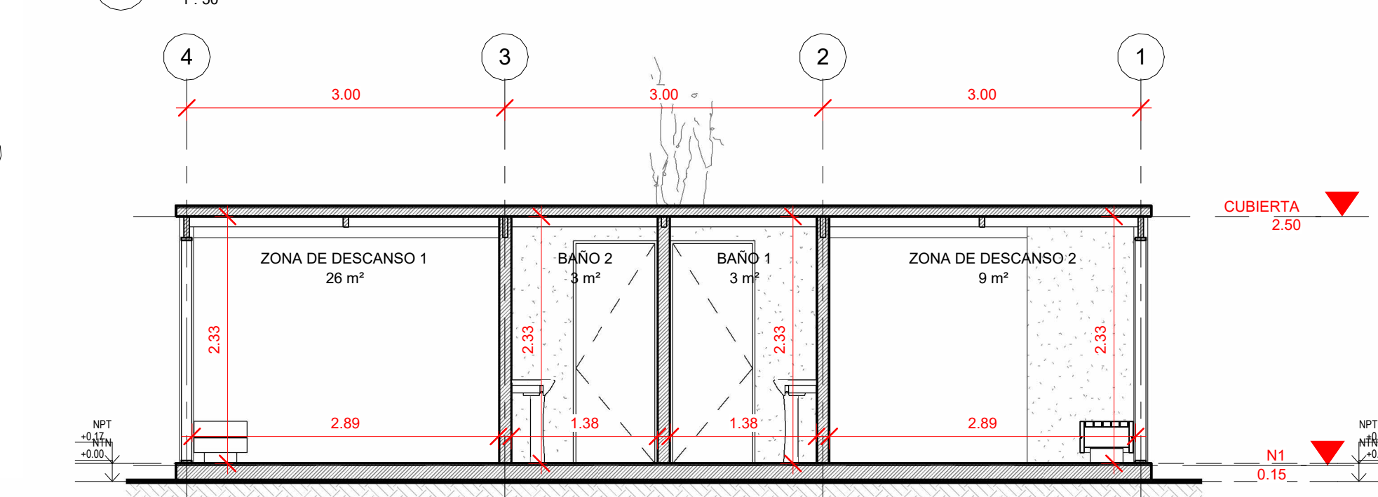
6 CORTE A 1 : 50
