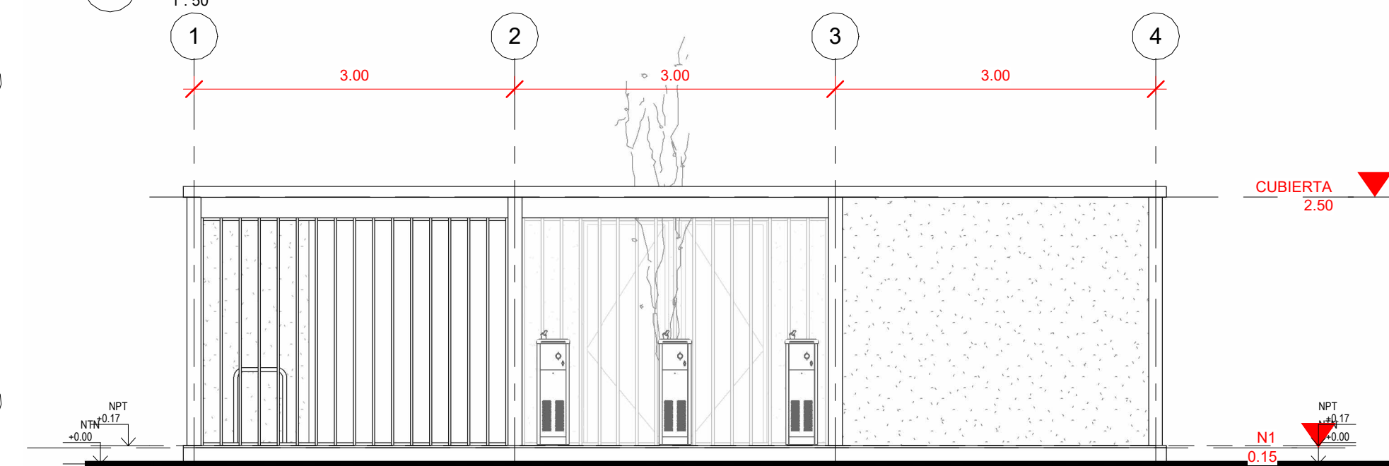
5 ELEVACIÓN 4 1 : 50
