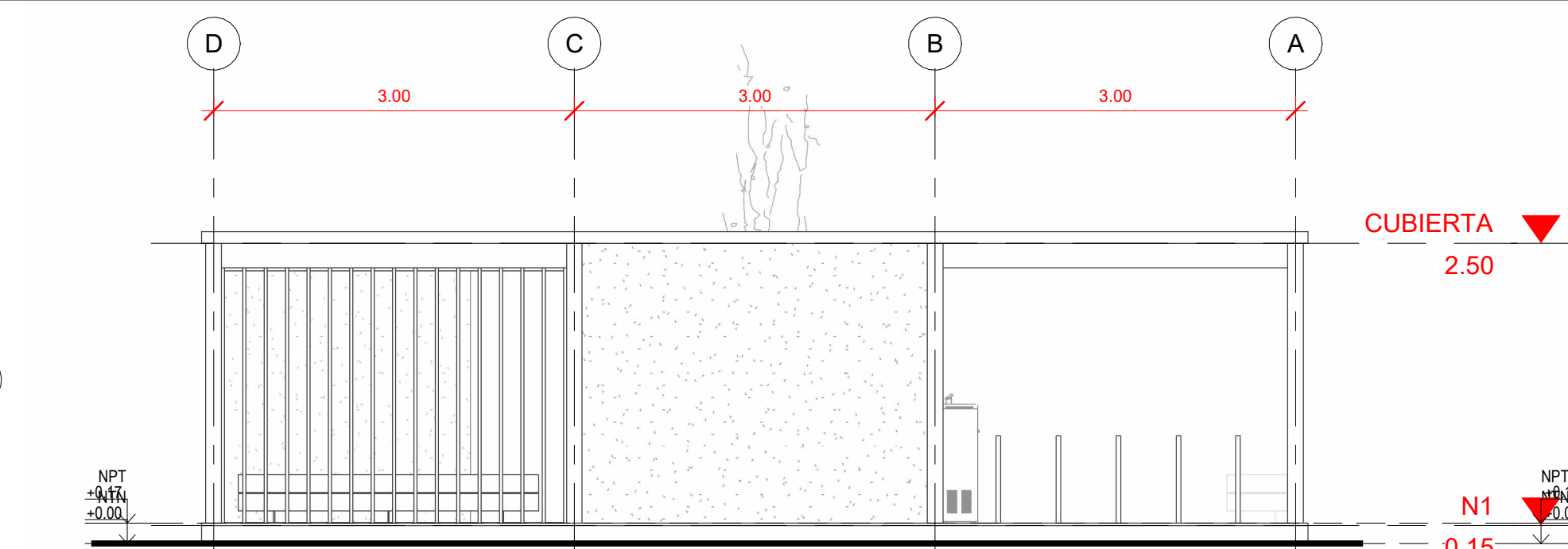
4 ELEVACIÓN 3 1:50
