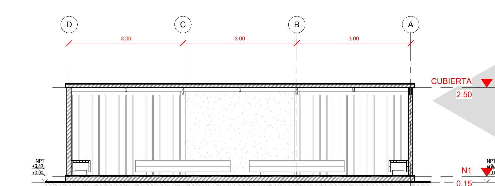
8 CORTE C 1:50
