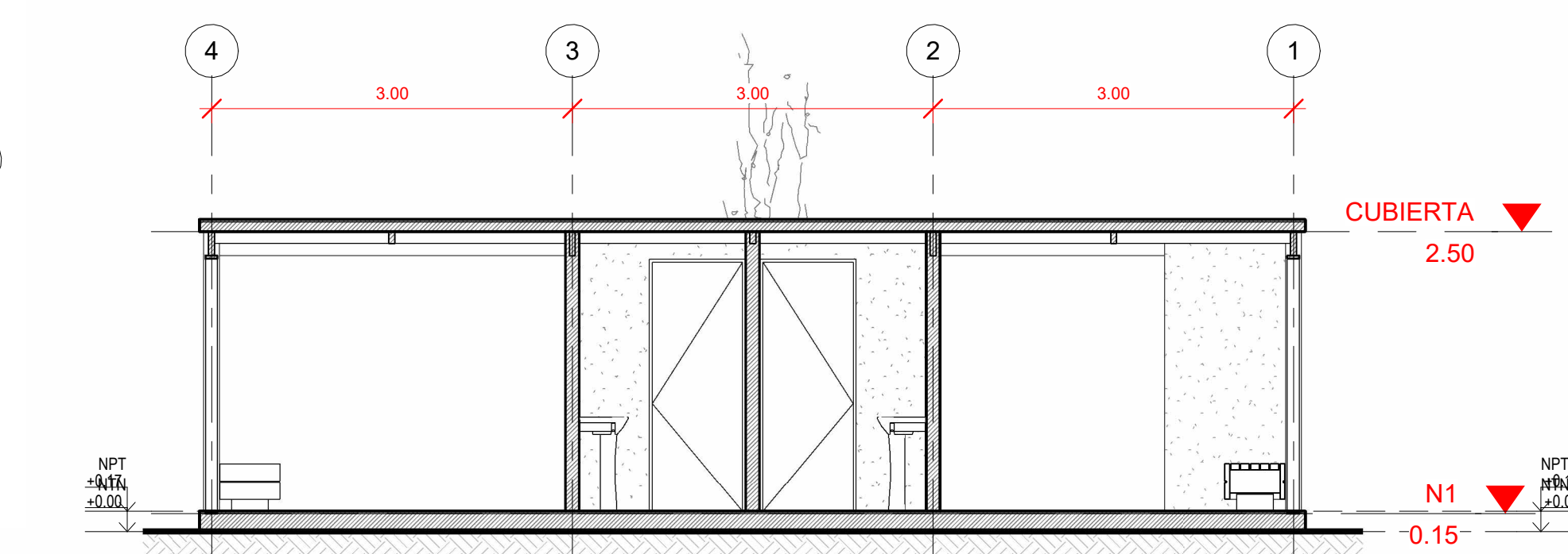
6 CORTE A 1:50
