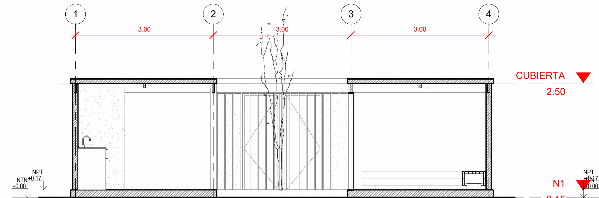
9 CORTE B 1:50
