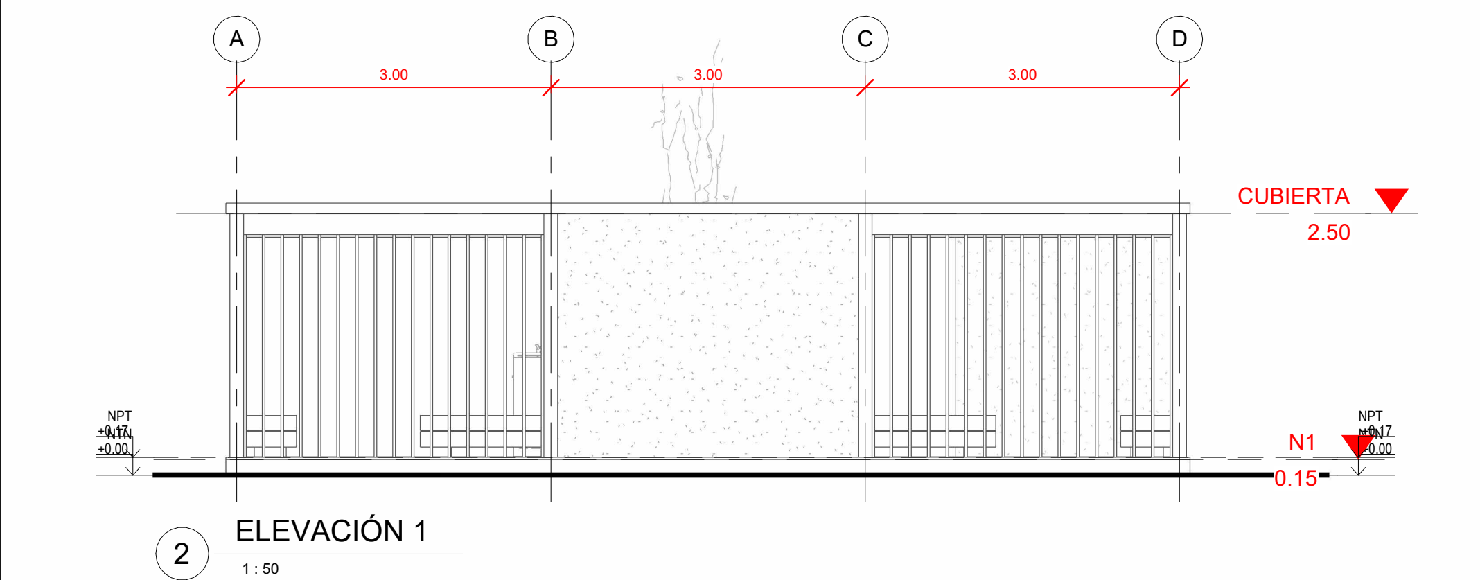
2 ELEVACIÓN 1 1:50
