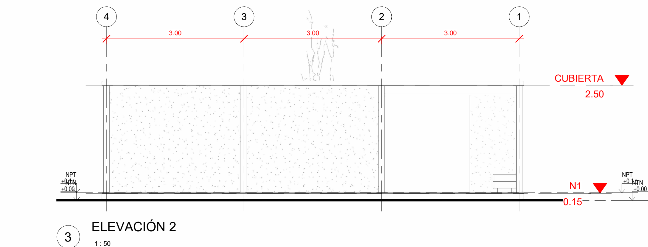
3 ELEVACIÓN 2 1:50
