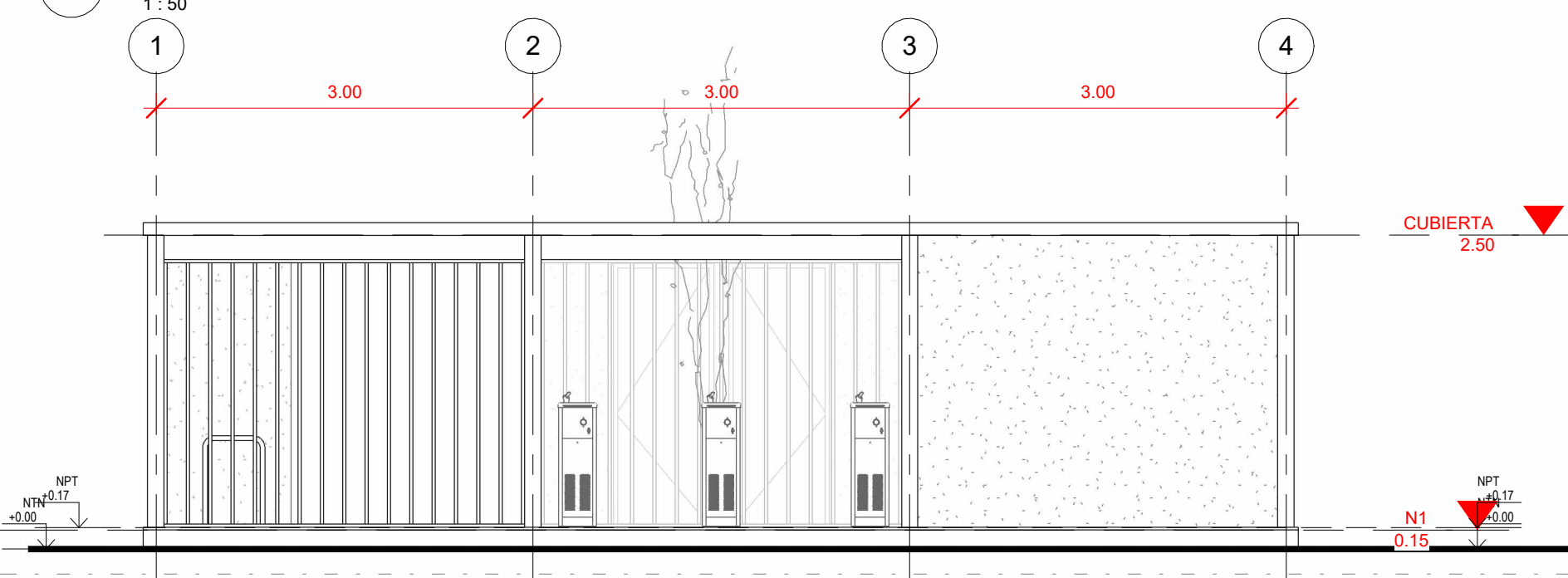
5 ELEVACIÓN 4 1:50
