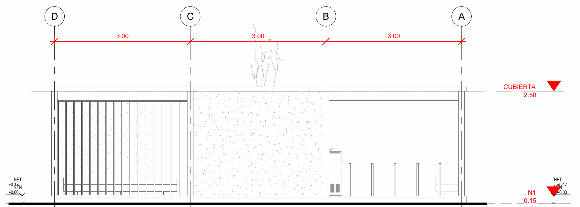
4 ELEVACIÓN 3 1:50
