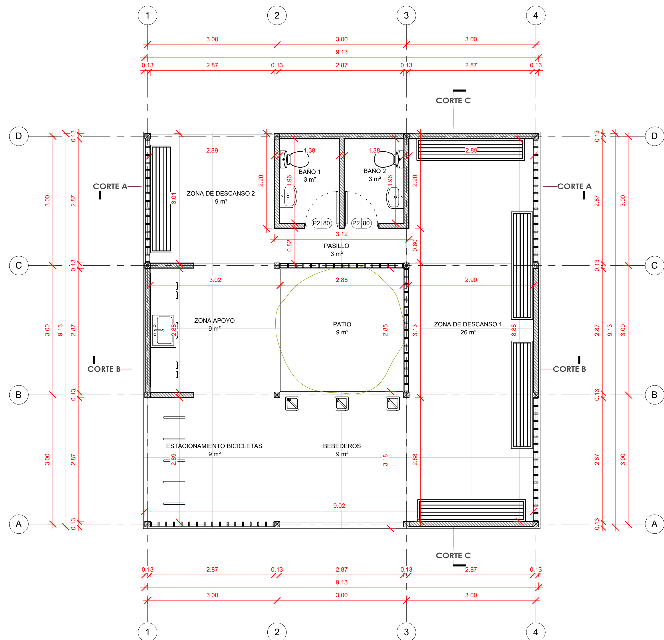
1 PLANTA DE ARQUITECTURA 1:50
