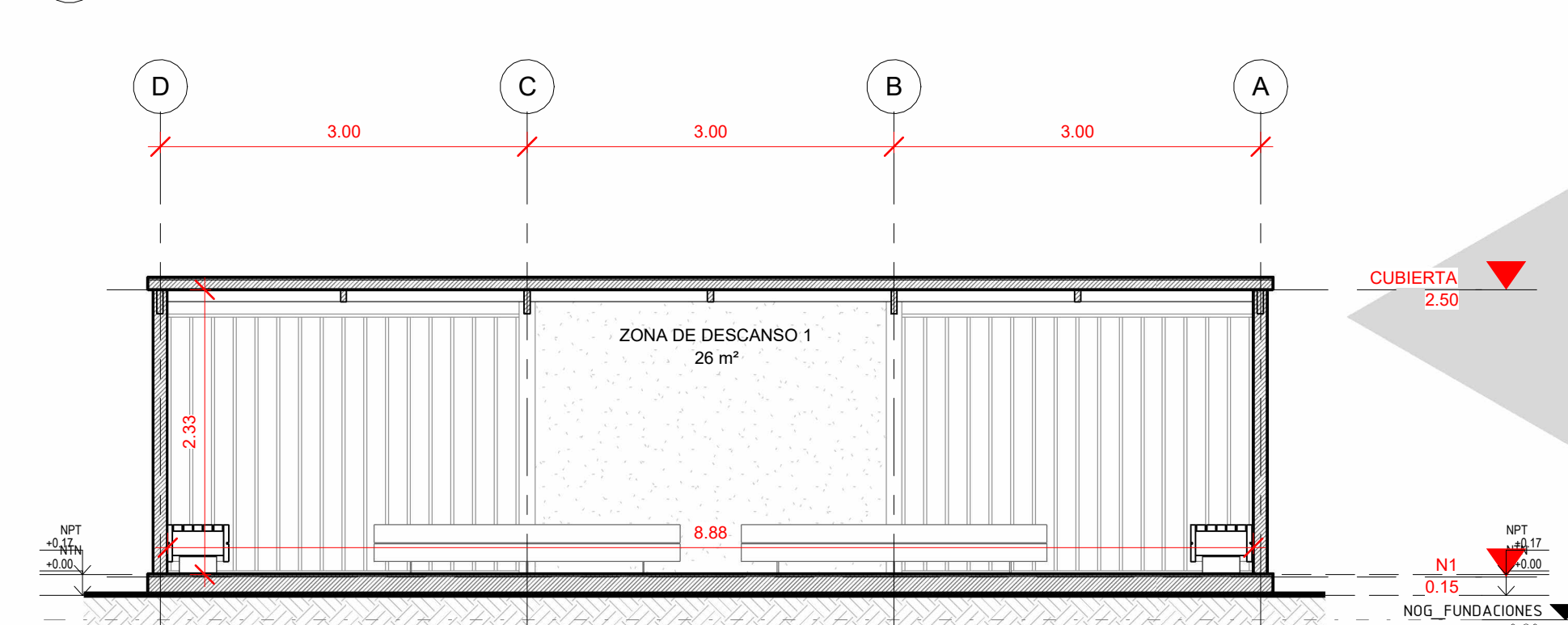
8 CORTE C 1:50
