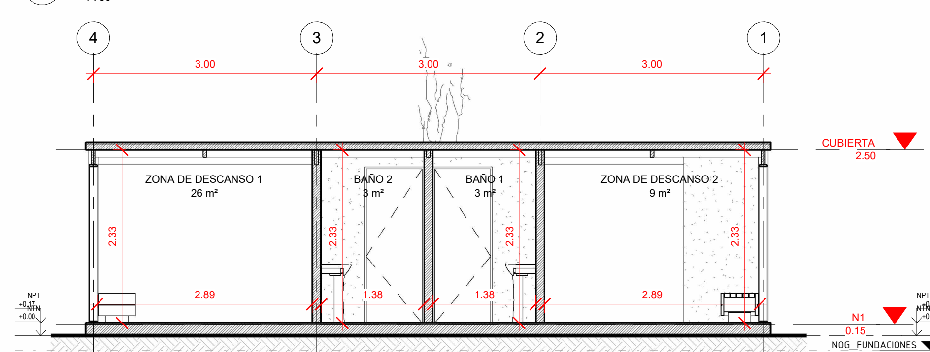
6 CORTE A 1:50
