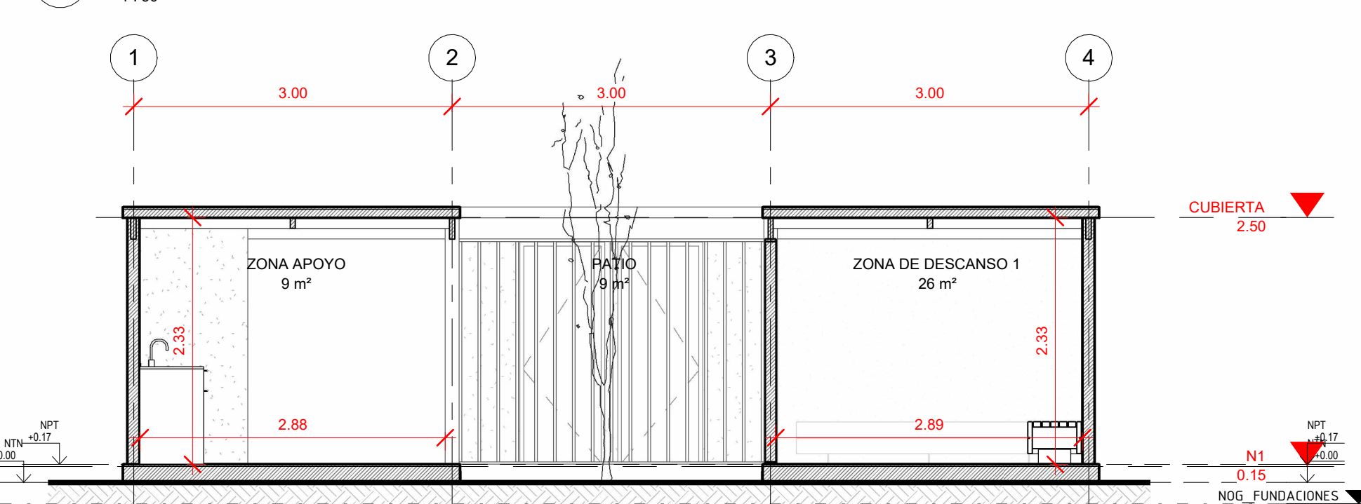
9 CORTE B 1:50
