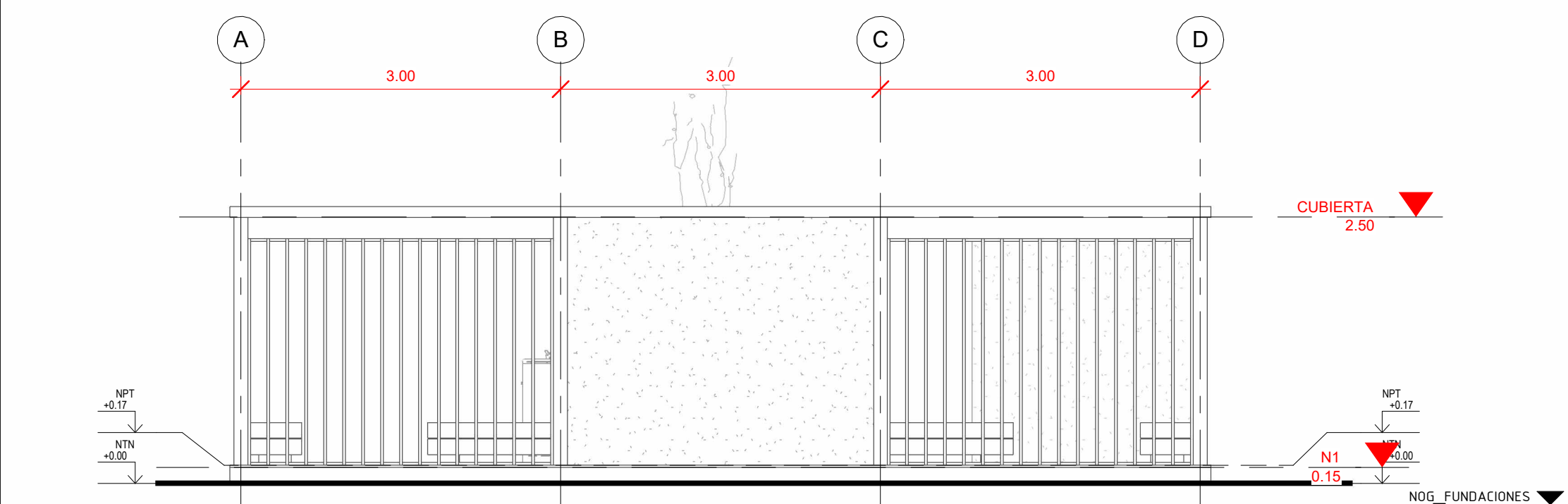
2 ELEVACIÓN 1 1 : 50
