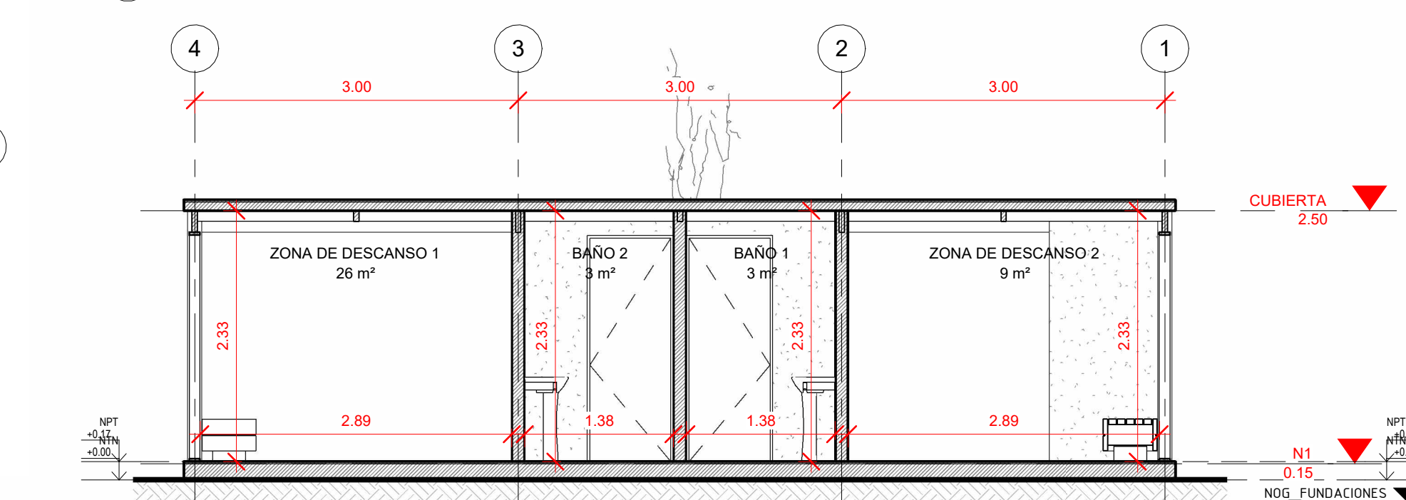
6 CORTE A 1 : 50
