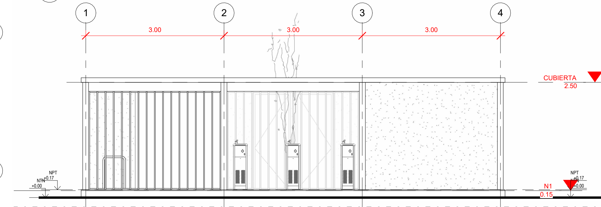
5 ELEVACIÓN 4 1 : 50
