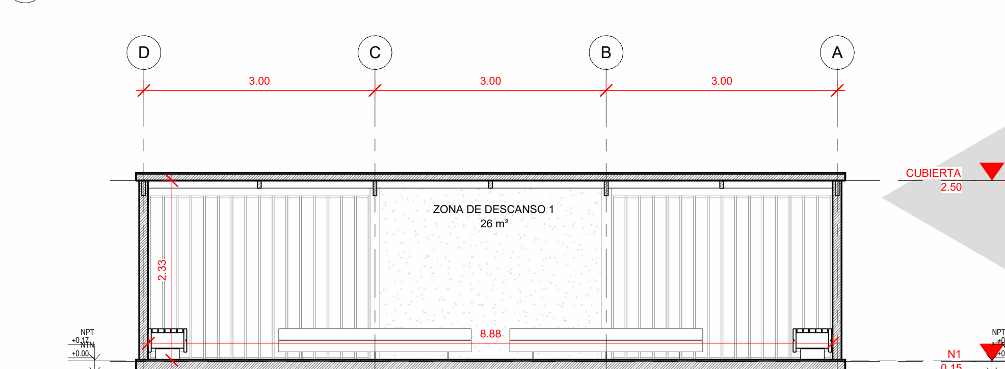
8 CORTE C 1 : 50
