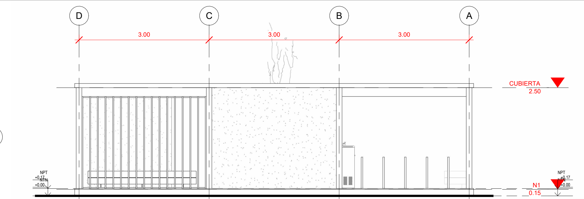
4 ELEVACIÓN 3 1 : 50
