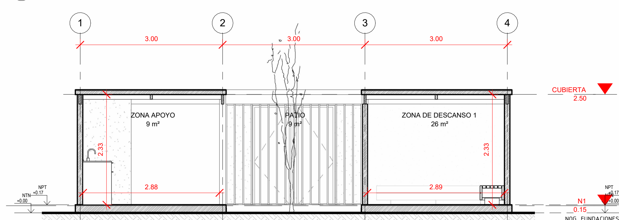
9 CORTE B 1 : 50
