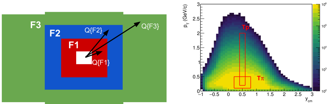
Рис. 12 — Слева: Схема разделения модулей FHCAL по группам для определения плоскости симметрии события. Справа: Кинематические окна для подсчета Q_1 -векторов из треков заряженных частиц.
