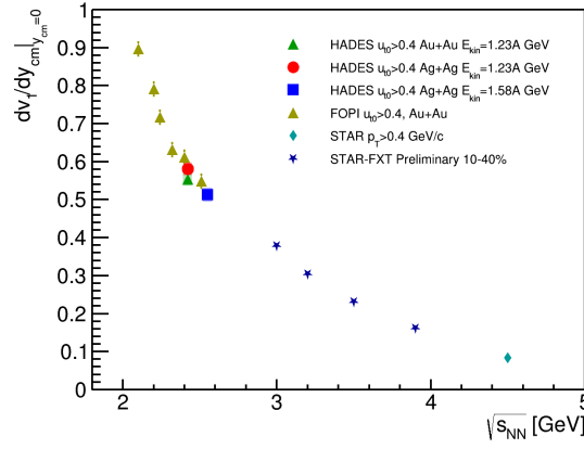
Рис. 10 — Зависимость dv_1/dy|_{y_{cm}=0} протонов в среднецентральных столкновениях от энергии столкновения \sqrt{s_{NN}} .
