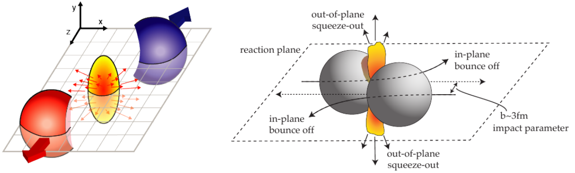
Рис. 1 — Схематическое изображение механизмов происхождения направленного v_1 и эллиптического v_2 потоков в столкновениях ядер при энергиях \sqrt{s_{NN}} > 25 ГэВ (слева) и \sqrt{s_{NN}} = 2-4 ГэВ (справа).
