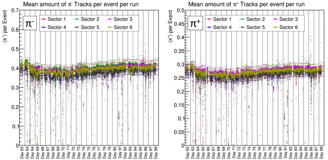
Рисунок 3.4 — Среднее число отрицательно (слева) и положительно заряженных (справа) пионов в событии в зависимости от дня набора данных для столкновений \text{Ag} + \text{Ag} при E_{kin} = 1.58A ГэВ. Маркерами различных цветов обозначены сектора установки HADES, в который производился подсчет.
