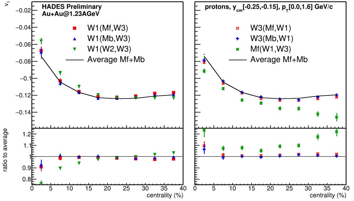
Рисунок 3.16 — Зависимость направленного потока протонов v_1 от центральности в столкновениях Au+Au при энергии E_{kin} = 1.23A ГэВ.
