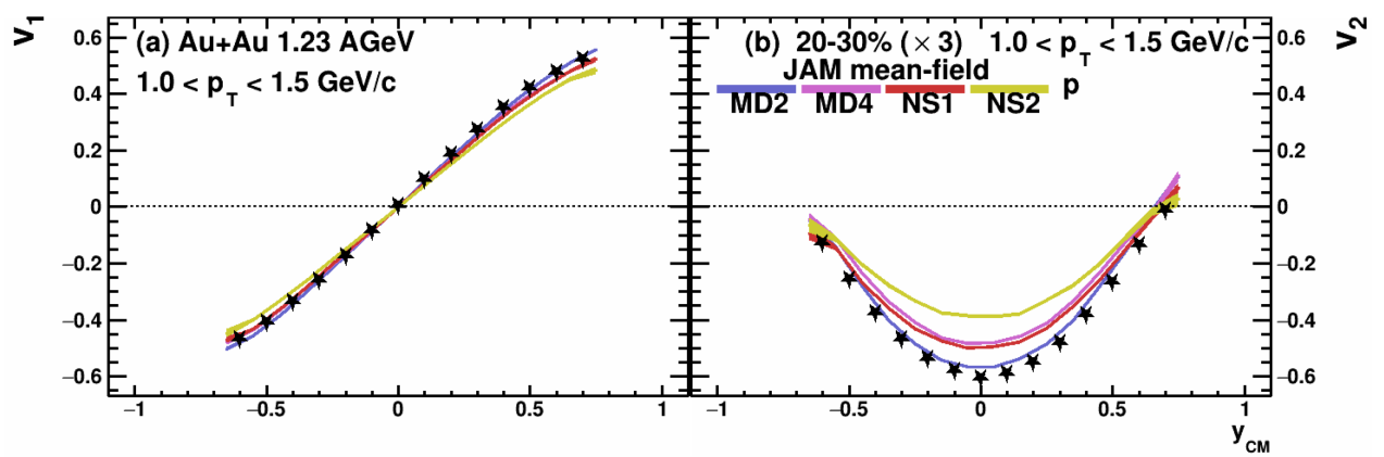
Рисунок 3.21 — Сравнение экспериментальных значений v_1 и v_2 с теоретическими предсказаниями модели JAM с различными потенциалами.
