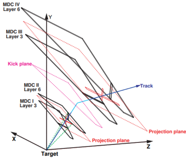
Рисунок 2.3 — Схематическое изображение трекингowej системы эксперимента HADES.
