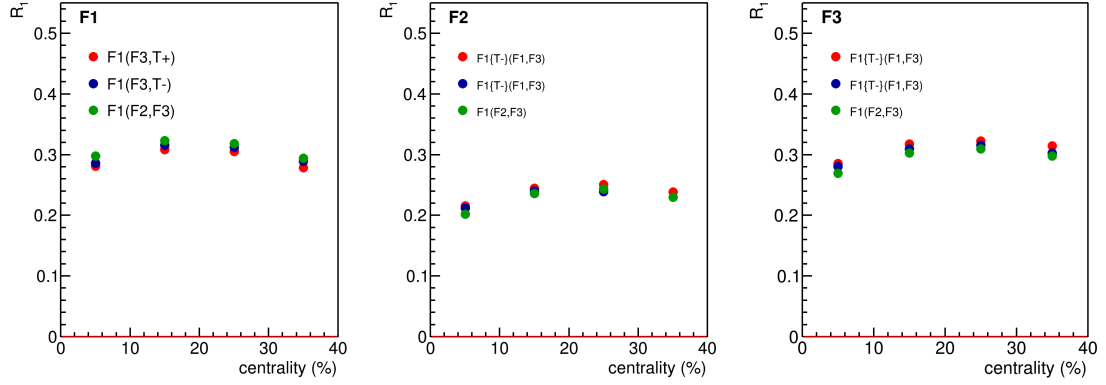
Рис. 12 — Зависимость разрешения плоскостей симметрии F1 , F2 и F3 от центральности из анализа экспериментальных данных BM@N для столкновений Xe+Cs(I) при энергии E_{\text{kin}} = 3,8\text{A} ГэВ [A9].
