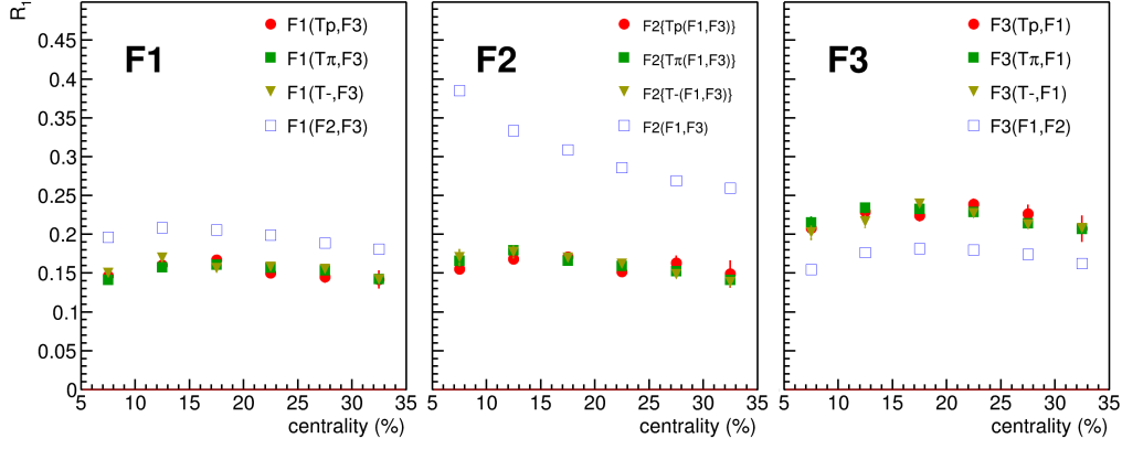
Рис. 11 — Зависимость разрешения R_1 плоскостей симметрии F1 – F3 от центральности для различных комбинаций \mathbf{Q}_1 -векторов [A3; A4; A6].
