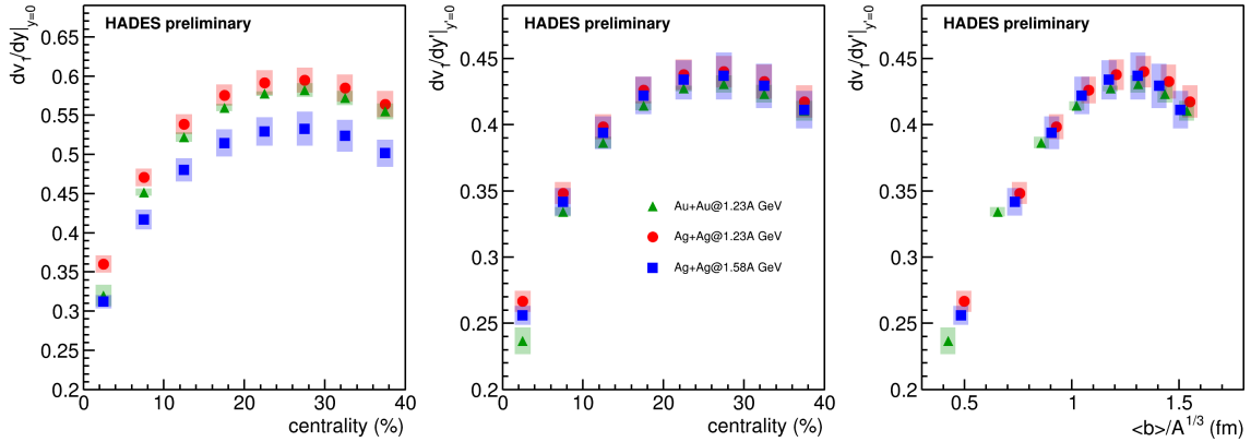
Рис. 14 — Зависимость dv_1/dy|_{y=0} протонов от центральности: для y = y_{cm} (слева), для y_{cm} , номированной на быстроту пучка, y' = y_{cm}/y_{beam} (в центре) и для dv_1/dy'|_{y'=0} как функции \langle b \rangle / A^{1/3} (справа) [A4; A7; A8].
