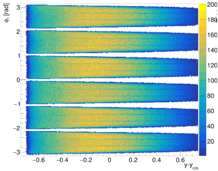
Рисунок 3.12 — Азимутальный акцептанс трекинговой системы эксперимента NADES в зависимости от быстроты частицы.
