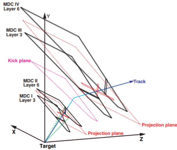
Рисунок 2.3 — Схмееатическое изображение трекинговой системы эксперимента HADES.
