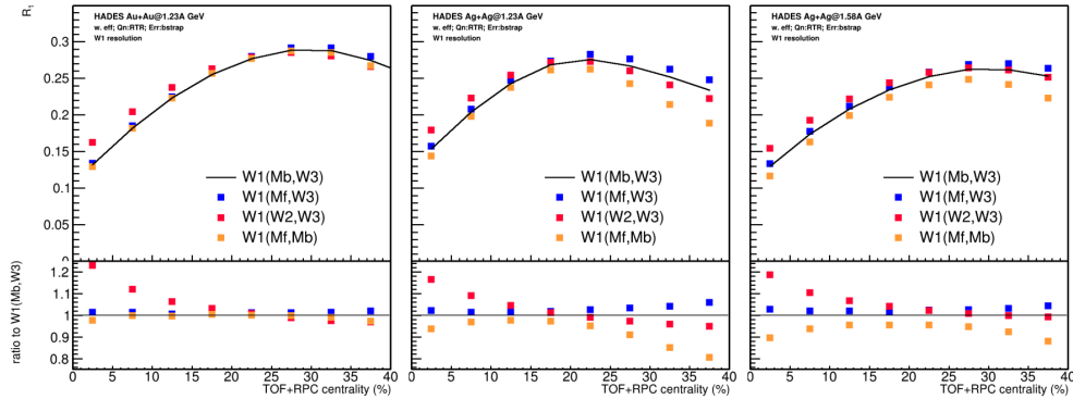
Рисунок 3.11 — Сравнение разрешений плоскости симметрии W1 полученное с использованием различных комбинаций Q_1 -векторов для \text{Au}+\text{Au}@1.23\text{A} ГэВ (слева), \text{Ag}+\text{Ag}@1.23\text{A} ГэВ (посередине) и \text{Ag}+\text{Ag}@1.58\text{A} ГэВ (справа)
