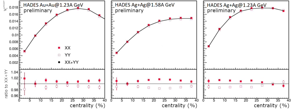
Рисунок 3.14 — Сравнение компонент корреляции \langle u_1 Q_1 \rangle после применения поправок на азимутальную неоднородность детектора для столкновений Au+Au@1.23A ГэВ (слева), Ag+Ag@1.23A ГэВ (посередине) и Ag+Ag@1.58A ГэВ (справа)
