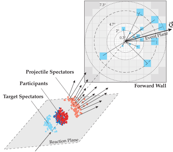
Рисунок 1.11 — Схематическое изображение распределения сигнала в модулях детектора Forward Wall, регистрирующего спектаторные фрагменты, летящие в плоскости реакции.
