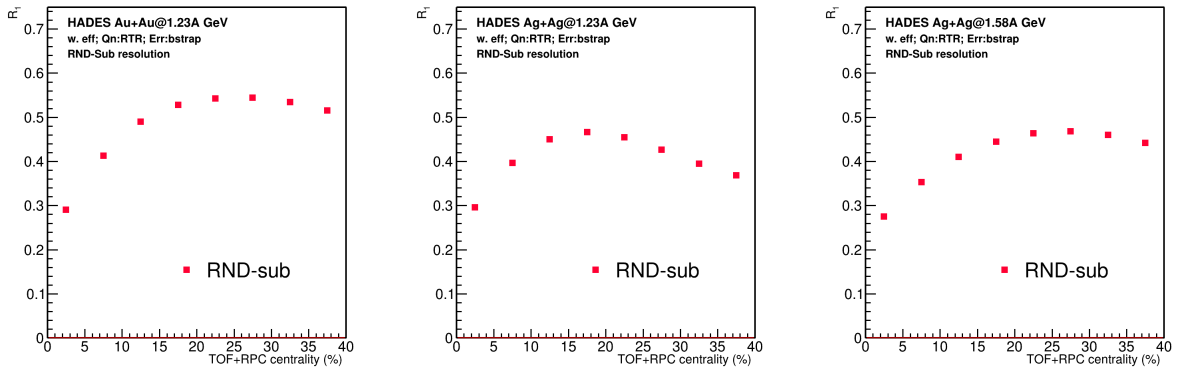
Рисунок 3.10 — Зависимость разрешение плоскости симметрии рассчитанное методом случайных подсобытий от центральности столкновения. Слева: для столкновений Au + Au при E_{kin}=1.23A ГэВ; посередине: для столкновений Ag + Ag при E_{kin}=1.23A ГэВ; справа: для столкновений Ag + Ag при E_{kin}=1.58A ГэВ;
