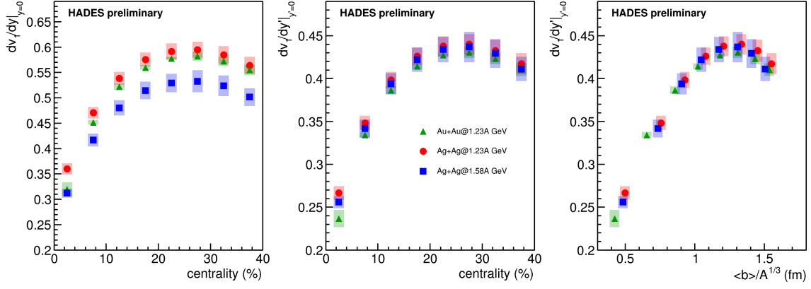
Рис. 10 — Зависимость dv_1/dy|_{y=0} протонов от центральности: (слева) для y = y_{cm} , (в центре) для y_{cm} номированной на быстроту пучка y' = y_{cm}/y_{beam} и (справа) для dv_1/dy'|_{y'=0} как функции \langle b \rangle нормированного на A^{1/3} [A4—A6].
