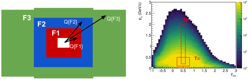
Рис. 11 — Слева: Схема разделения модулей FCHal по группам для определения плоскости симметрии события. Справа: Кинематические окна для подсчета Q_1 -векторов из треков заряженных частиц [A6—A8].
