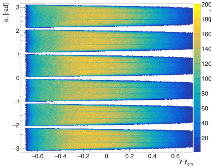
Рисунок 3.10 — Азимутальный аксептанс трекинговой системы эксперимента NADES в зависимости от быстроты частицы.
