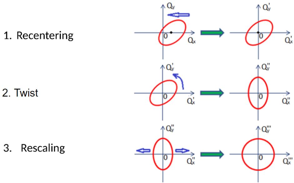
Рисунок 3.11 — Схематическое изображение поправок предложенных в [66].
