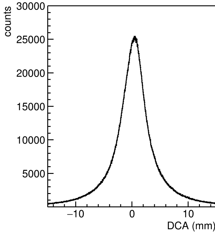
Рисунок 3.2 — Распределение восстановленных траекторий заряженных частиц по расстоянию наименьшего сближения с вершиной столкновения для \text{Au} + \text{Au} при E_{kin} = 1.23A ГэВ.
