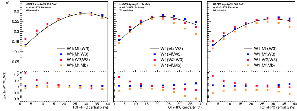
Рисунок 3.14 — Сравнение разрешений плоскости симметрии W1 полученное с использованием различных комбинаций Q_1 -векторов для Au+Au@1.23A ГэВ (слева), Ag+Ag@1.23A ГэВ (посередине) и Ag+Ag@1.58A ГэВ (справа)
