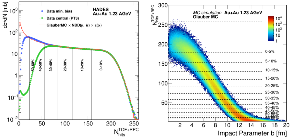
Рисунок 3.4 — Слева: распределение множественности срабатываний системы TOF-RPC в сеансе Au + Au при энергии 1.23A ГэВ. Справа: распределение разыгранной множественности методом МК-Глаубера и прицельного параметра для столкновений Au + Au при энергии 1.23A ГэВ.
