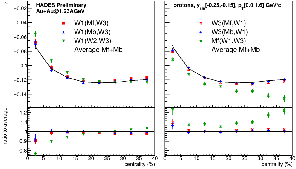
Рисунок 3.15 — Направленный поток протонов v_1 рожденных в столкновении Au+Au при энергии E_{kin}=1.23A ГэВ как функция центральности столкновения, измеренный при помощи различных комбинаций Q_1 -векторов.
