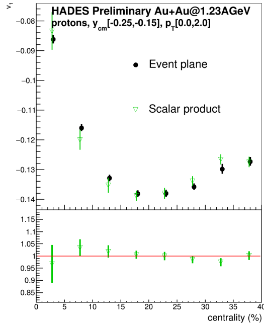
Рисунок 3.16 — Направленный поток протонов v_1 , рожденных в столкновении Au+Au при энергии E_{kin}=1.23A ГэВ как функция центральности столкновения. Результаты показаны для методов скалярного произведения (SP) и плоскости события (EP).
