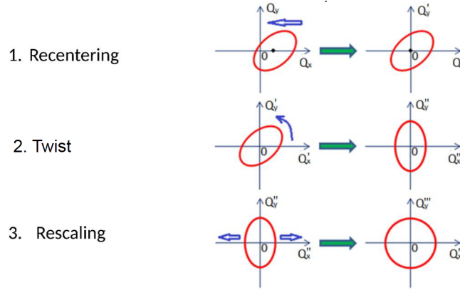
Рисунок 1.10 — Схематическое представление эффекта применения каждого этапа коррекций, описанных в [66].
