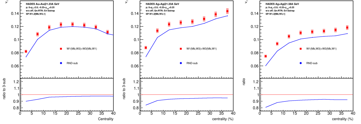
Рисунок 3.17 — Направленный поток v_1 протонов, рожденных в столкновении Au+Au при энергии E_{kin} = 1.23A ГэВ (слева), Ag + Ag при энергии E_{kin} = 1.23A ГэВ (посередине) и Ag + Ag при энергии E_{kin} = 1.58A ГэВ (справа) как функция центральности столкновения. Результаты показаны для методов трех подсобытий и метода случайных подсобытий.
