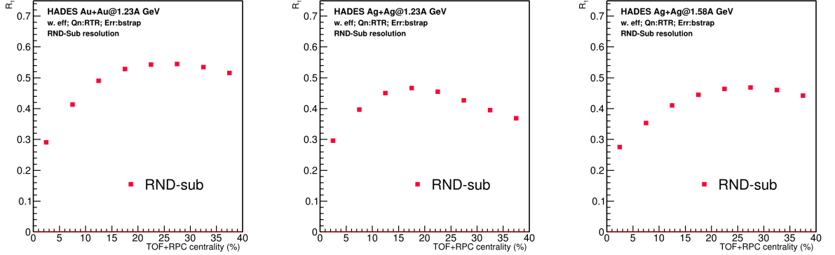
Рисунок 3.13 — Разрешение плоскости симметрии рассчитанное методом случайных подсобытий как функция центральности столкновения. Слева: для столкновений Au + Au при E_{kin}=1.23A ГэВ; посередине: для столкновений Ag + Ag при E_{kin}=1.23A ГэВ; справа: для столкновений Ag + Ag при E_{kin}=1.58A ГэВ;
