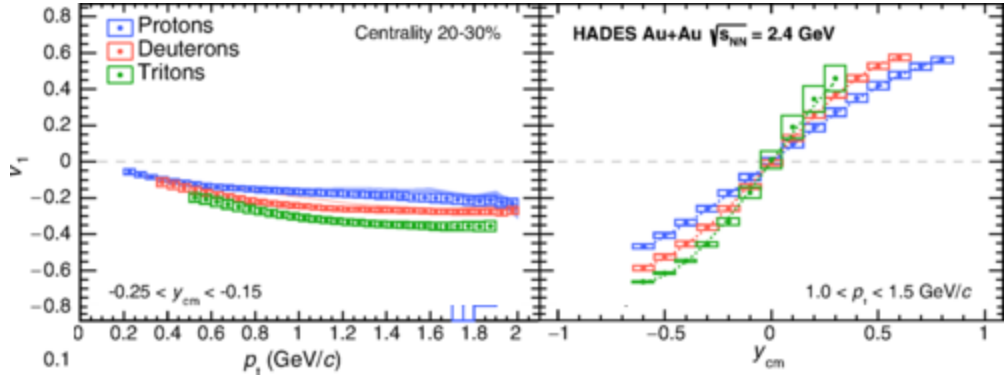
Рисунок 4.1 — Направленный поток ( v_1 ) протонов, дейтронов и тритонов рожденных в столкновении Au+Au при энергии E_{kin}=1.23A ГэВ как функция быстроты (справа) и поперечного импульса (слева).
