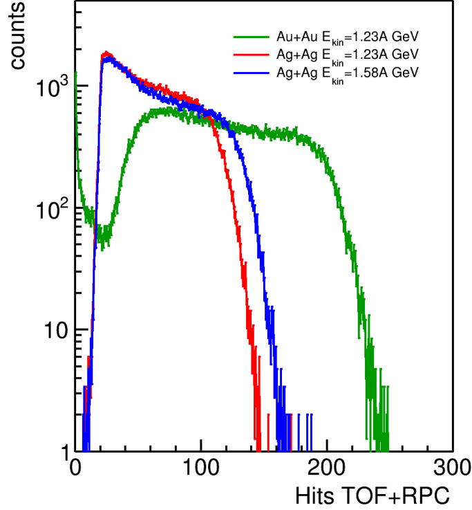
Рисунок 3.3 — Сравнение множественности срабатываний времяпролётной системы TOF+RPC для центрального триггера в столкновениях Au + Au при E_{kin} = 1.23 и Ag + Ag при E_{kin} = 1.23 и E_{kin} = 1.58A ГэВ.
