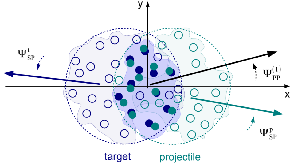
Рисунок 1.9 — Схематическое представление сталкивающихся ядер в плоскости, перпендикулярной направлению пучка.
