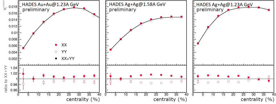
Рисунок 3.12 — Сравнение компонент корреляции \langle u_1 Q_1 \rangle после применения поправок на азимутальную неоднородность детектора для столкновений Au+Au@1.23A ГэВ (слева), Ag+Ag@1.23A ГэВ (посередине) и Ag+Ag@1.58A ГэВ (справа)
