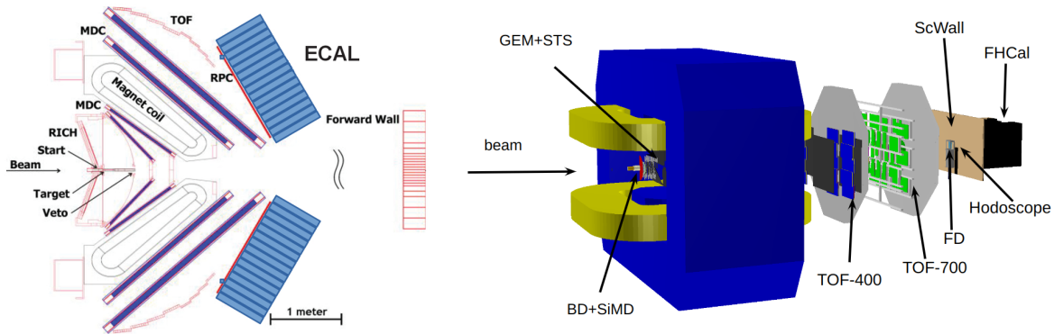
Рис. 2 — Схема экспериментов HADES [15] (слева) и BM@N [22] (справа).
