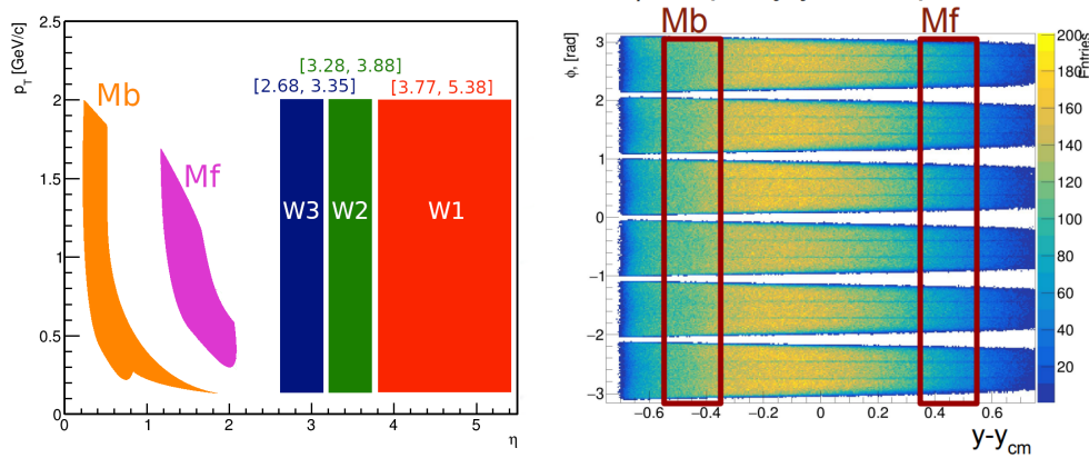
Рис. 4 — Схематическое изображение акцептанса p_T vs \eta , использованного для построения пяти \mathbf{Q}_1 -векторов для анализа v_1 протонов (слева). Азимутальный акцептанс протонов в плоскости \phi vs y_{cm} (справа) [A1].
