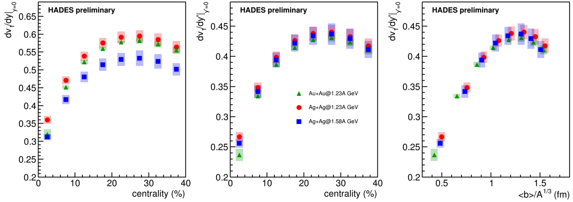
Рис. 14 — Зависимость dv_1/dy|_{y=0} протонов от центральности: для y = y_{cm} (слева), для y_{cm} , нормированной на быстроту пучка, y' = y_{cm}/y_{beam} (в центре) и для dv_1/dy'|_{y'=0} как функции \langle b \rangle/A^{1/3} (справа) [A4; A7; A8].
