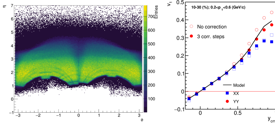
Рис. 10 — Азимутальный акцептанс трековой системы BM@N (слева). Сравнение v_1(y_{cm}) протонов в модельных столкновениях Xe+Cs(I) для x - и y -компонент \mathbf{u}_1 - и \mathbf{Q}_1 -векторов: XX и YY (справа) до и после коррекции на азимутальную неоднородность акцептанса детектора [A3; A4; A6].
