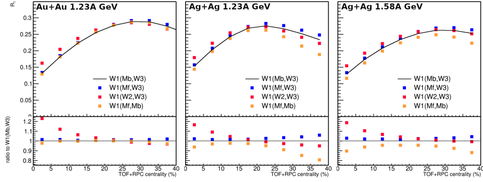
Рис. 6 — Зависимость разрешения R_1 от центральности для различных комбинаций \mathbf{Q}_1 -векторов для Au+Au и Ag+Ag столкновений [A7; A8].
