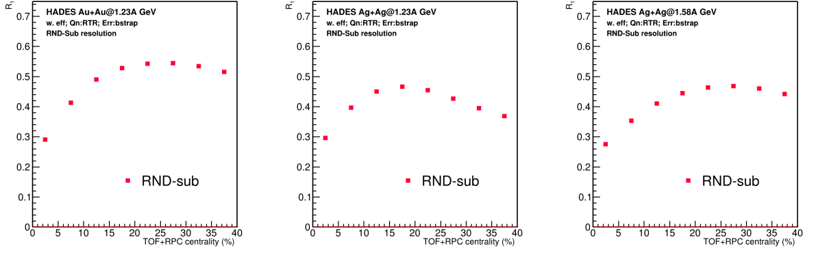
Рисунок 3.11 — Зависимость разрешение плоскости симметрии рассчитанное методом случайных подсобытий от центральности столкновения. Слева: для столкновений Au + Au при E_{kin}=1.23A ГэВ; посередине: для столкновений Ag + Ag при E_{kin}=1.23A ГэВ; справа: для столкновений Ag + Ag при E_{kin}=1.58A ГэВ;
