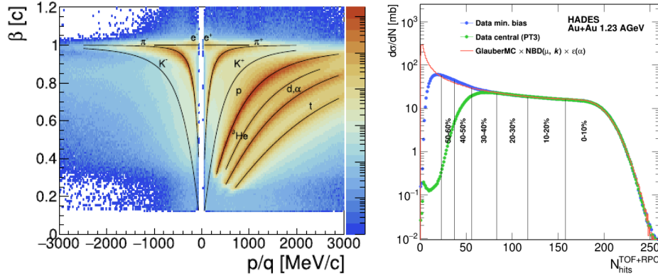
Рис. 3 — Слева: распределение частиц со скоростью \beta в зависимости от импульса частицы к заряду ( p/q ). Справа: распределение суммарной множественности хитов в системе МЕТА [25].
