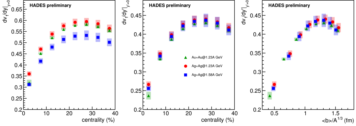
Рис. 14 — Зависимость dv_1/dy|_{y=0} протонов от центральности: (слева) для y = y_{cm} , (в центре) для y_{cm} номинированной на быстроту пучка y' = y_{cm}/y_{beam} и (справа) для dv_1/dy'|_{y'=0} как функции \langle b \rangle/A^{1/3} [A4; A7; A8].
