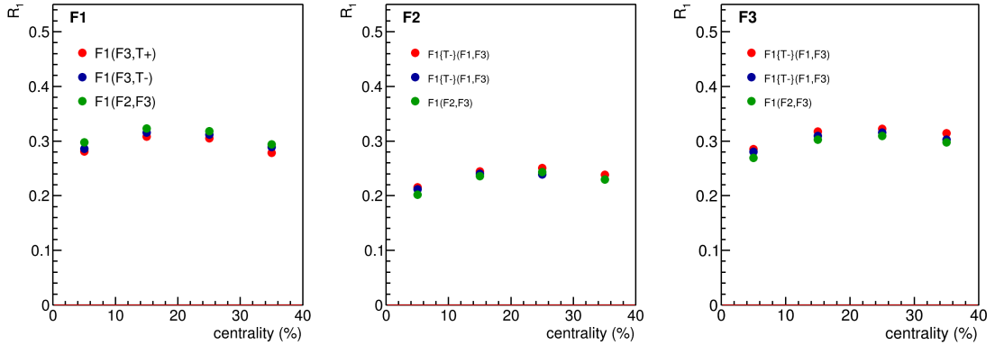
Рис. 12 — Зависимость разрешения плоскостей симметрии F1, F2 и F3 от центральности из анализа экспериментальных данных BM@N для столкновений Xe+Cs(I) при энергии E_{kin} = 3.8A ГэВ [A9].
