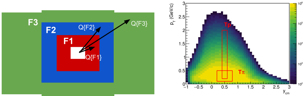
Рис. 9 — Схематическое изображение акцептанса для построения пяти Q_1 векторов из модулей FHCAL (слева) и треков частиц (справа) [A3; A4; A6].
