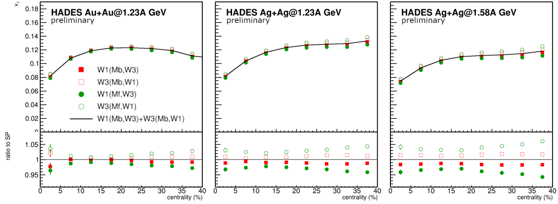
Рис. 7 — Зависимость v_1 протонов от центральности для различных комбинаций Q_1 -векторов для Au+Au и Ag+Ag столкновений [A7; A8].
