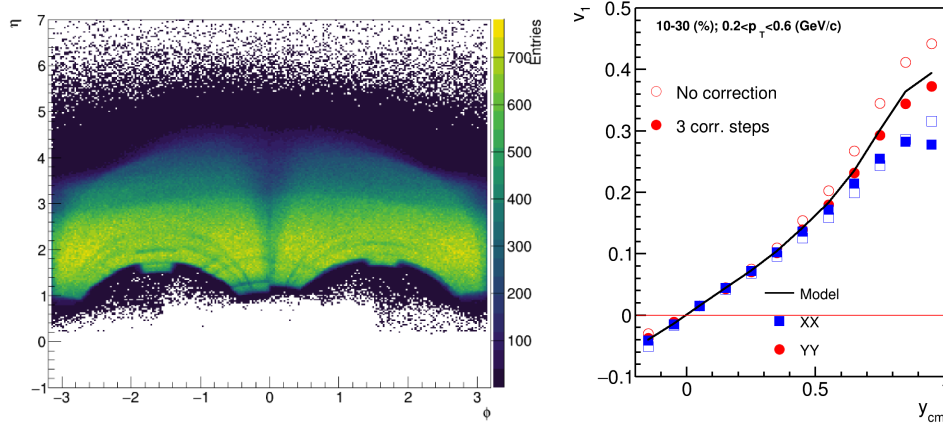
Рис. 10 — Азимутальный аксептанс трековой системы BM@N (слева). Сравнение v_1(y_{cm}) протонов в модельных столкновениях Xe+Cs(I) для x - и y - компонент u_1 и Q_1 векторов: XX и YY (справа) до и после коррекции на азимутальную неоднородность аксептанса детектора [A3; A4; A6].
