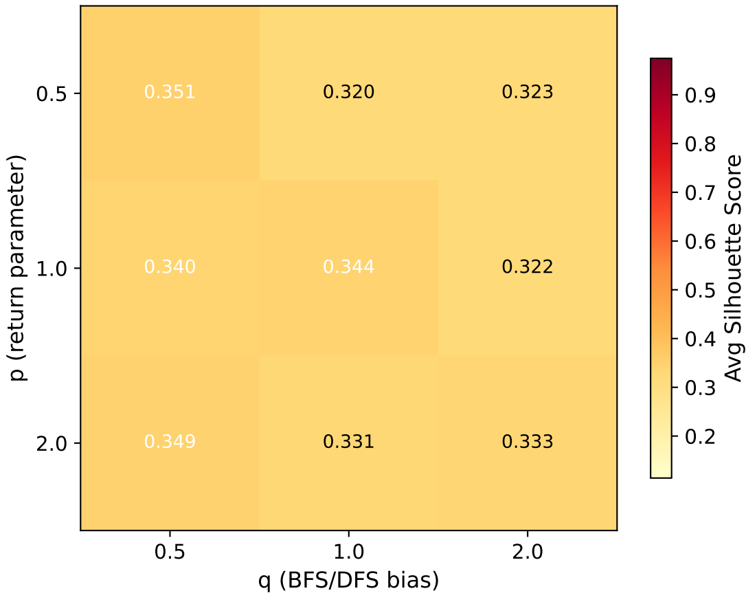
Node2Vec Sensitivity — d=5
