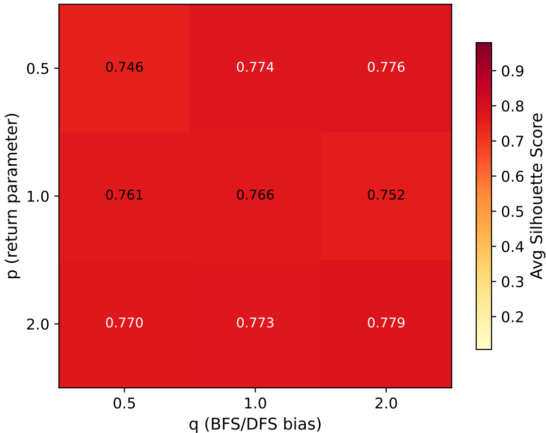
Node2Vec Sensitivity — d=1
