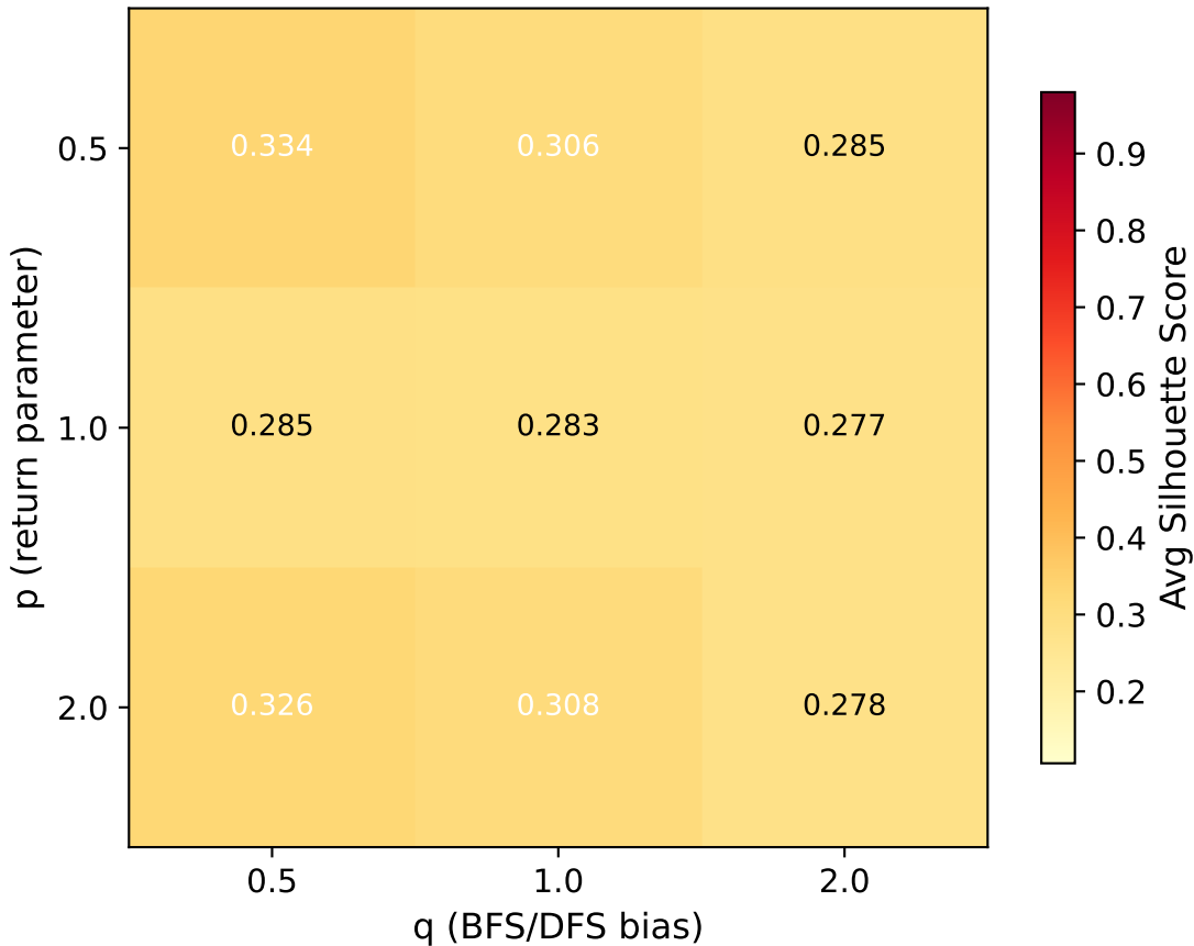
Node2Vec Sensitivity — d=10
