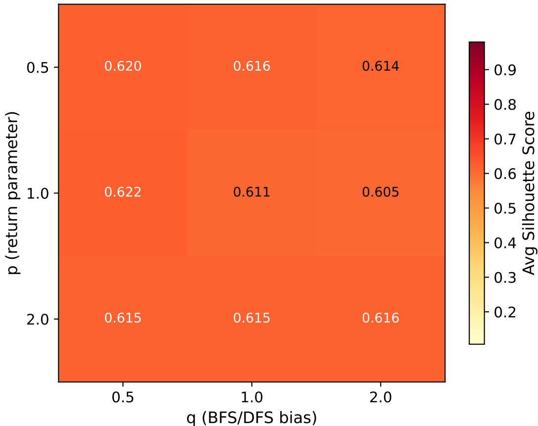
Node2Vec Sensitivity — d=2
