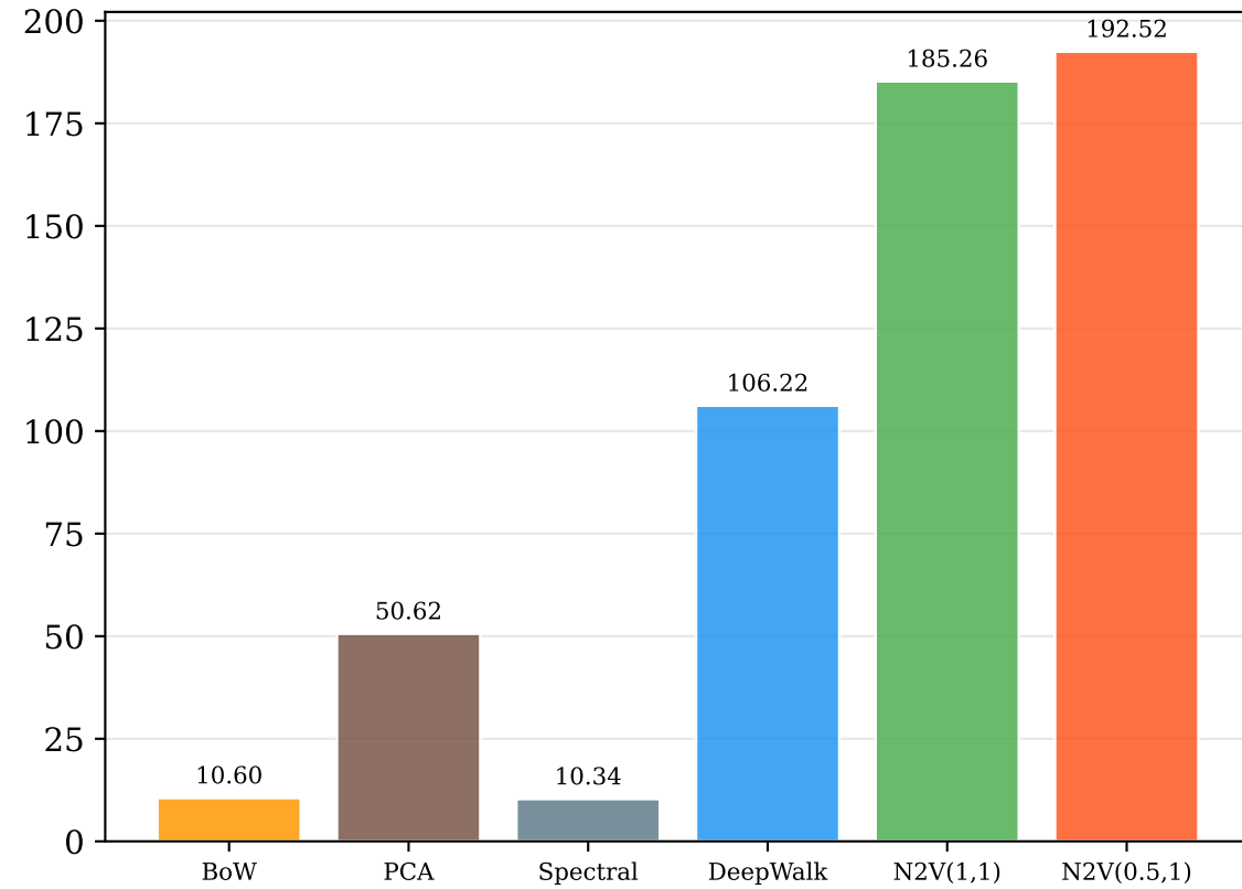
Calinski-Harabasz (↑)
