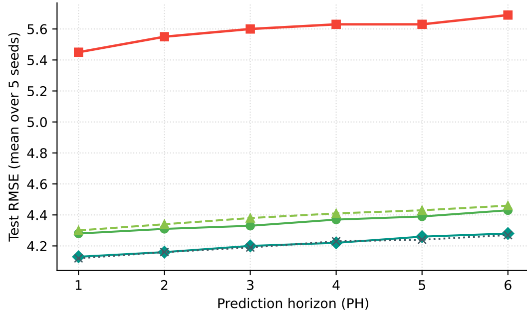
(b) SZ-Taxi (15 min)
