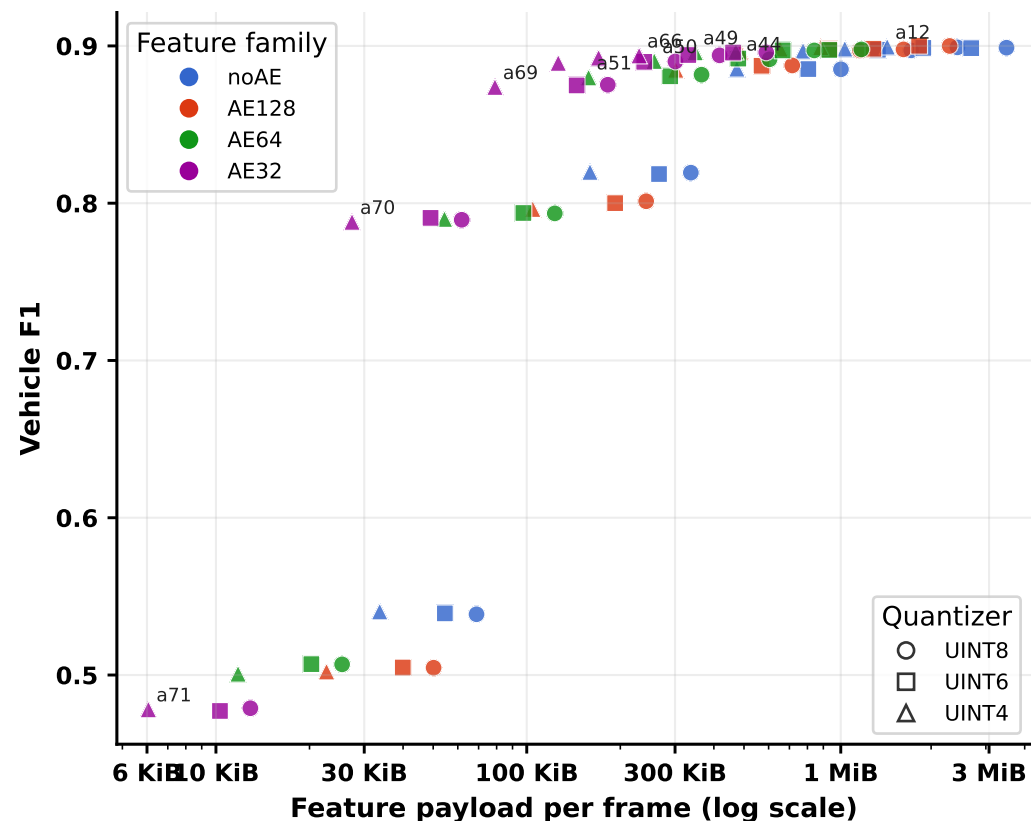
Vehicle detection F1
