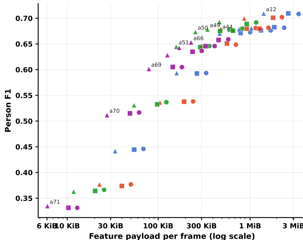
Person detection F1
