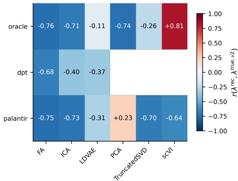
a v2 \lambda -correlation ( \sigma=0.3 )
