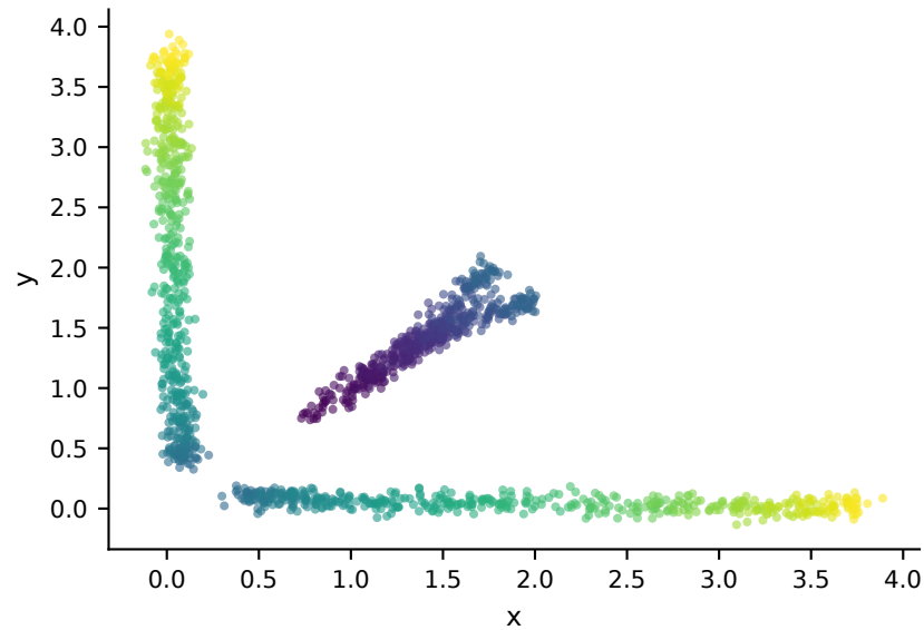
b v2 static interp
