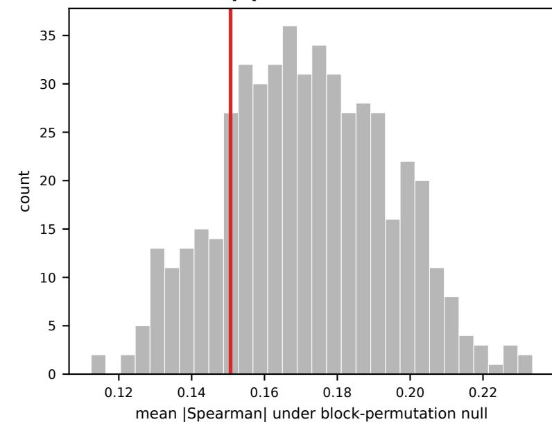
b M1 null (emp p=0.832)
