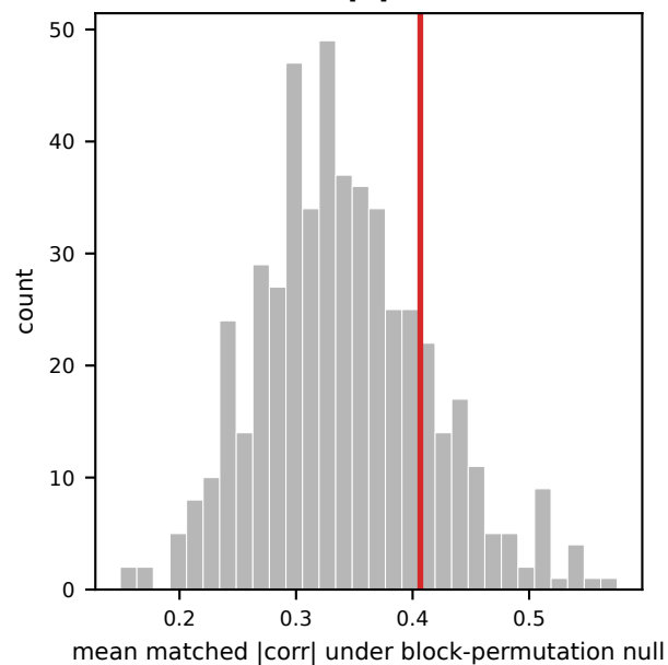
c M2 null (emp p=0.184)
