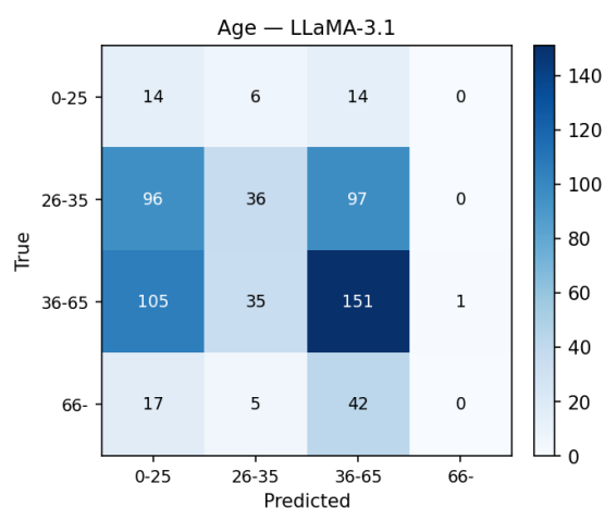
(d) LLaMA-3.1-8b
