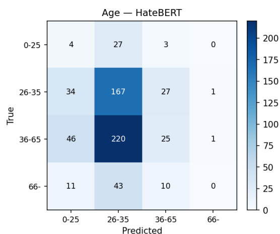
(b) HateBERT
