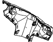
53206-KVB-T00ZC ฝาครอบแฮนด์ด้านหลัง
