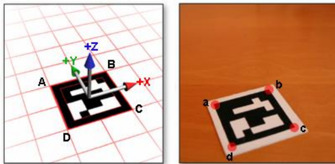
ภาพที่ 8.10 รูปซ้ายคือตัวอย่างการกำหนดพิกัด 3 มิติ ( X,Y,Z ) ของมาร์กเกอร์ในโลกเสมือน และรูปขวาคือพิกัด 2 มิติ ( x,y ) ของมาร์กเกอร์ที่พบจากภาพที่รับจากกล้องของระบบความเป็นจริงเสริม (ที่มา: https://www.researchgate.net/figure/216813818_fig1_Figure-2-Basic-workflow-of-an-AR-application-using-fiducial-marker-tracking และ https://www.google.com )
