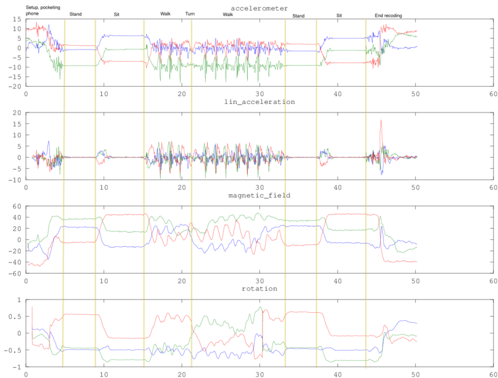
ภาพที่ 5.4 ตัวอย่างค่าที่อ่านได้จากเซ็นเซอร์วัดความเคลื่อนไหวในสมาร์ทโฟนระหว่างการทำกิจกรรมต่าง ๆ (ที่มา: http://rflasveld.github.io/blog/2013/04/12/visualizing-accelerometer-data/ และ https://www.google.com )
