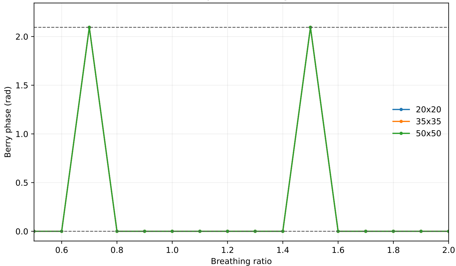
Z3 Berry Phase Convergence
