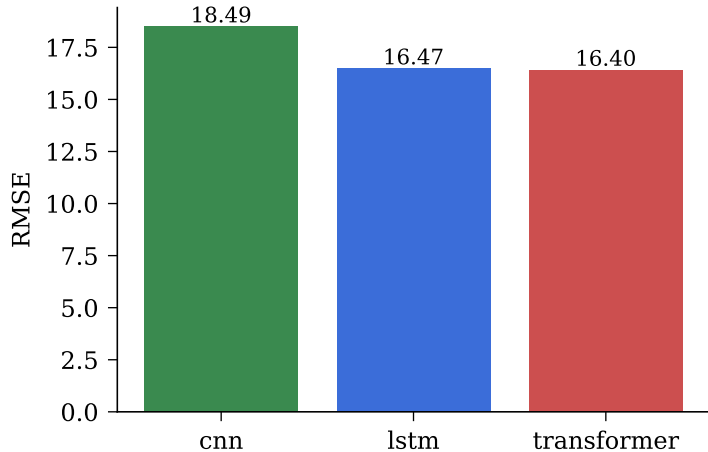
CMAPSS · Test RMSE
