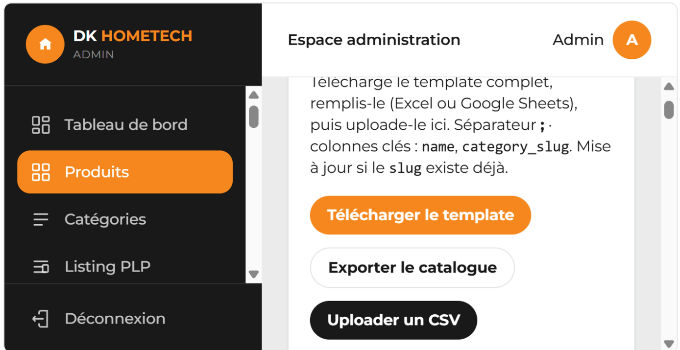
Figure 15 — Template, export du catalogue et upload. Le séparateur est le point-virgule.
