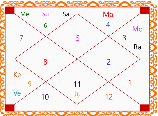
Shastiamsa Chart
