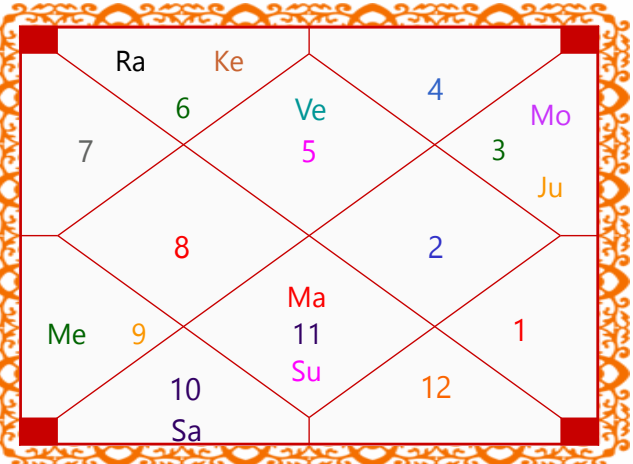
Khavedamsa Chart
