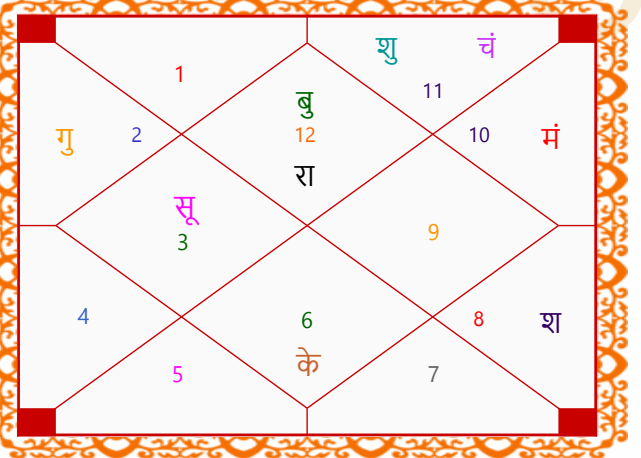
सप्तविंशांश कुंडली
