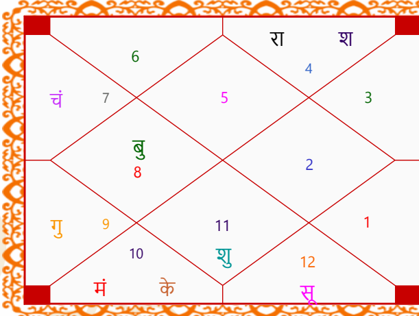
सप्तमांश कुंडली
