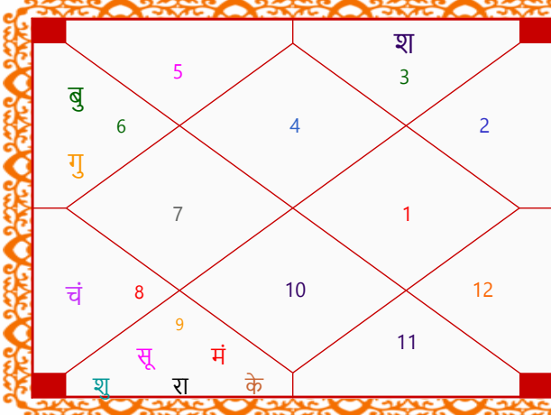
पंचमांश कुंडली
