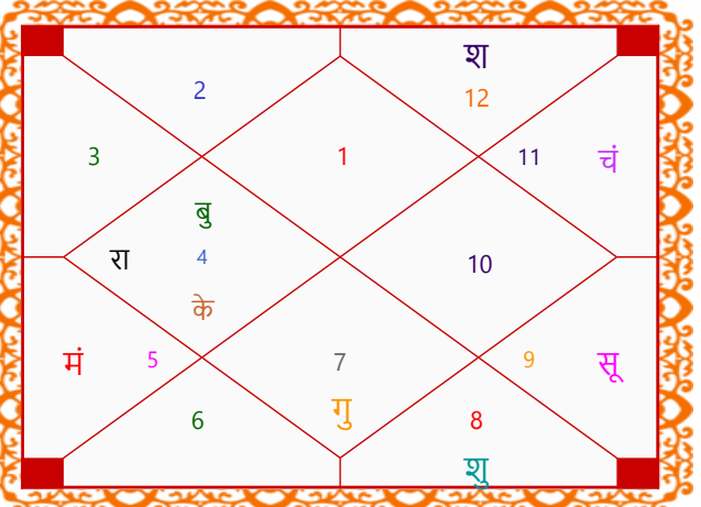
अष्टमांश कुंडली
