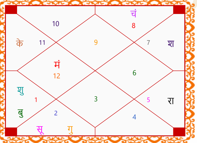
दशमांश कुंडली
