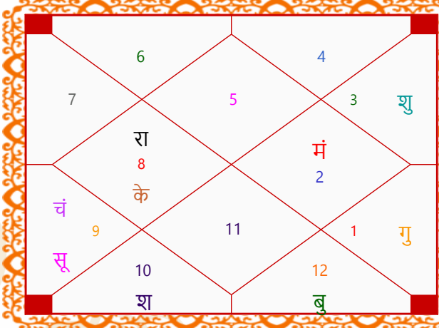
अक्षवेदांश कुंडली
