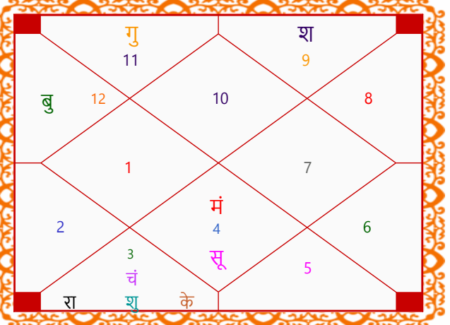
षष्ठांश कुंडली
