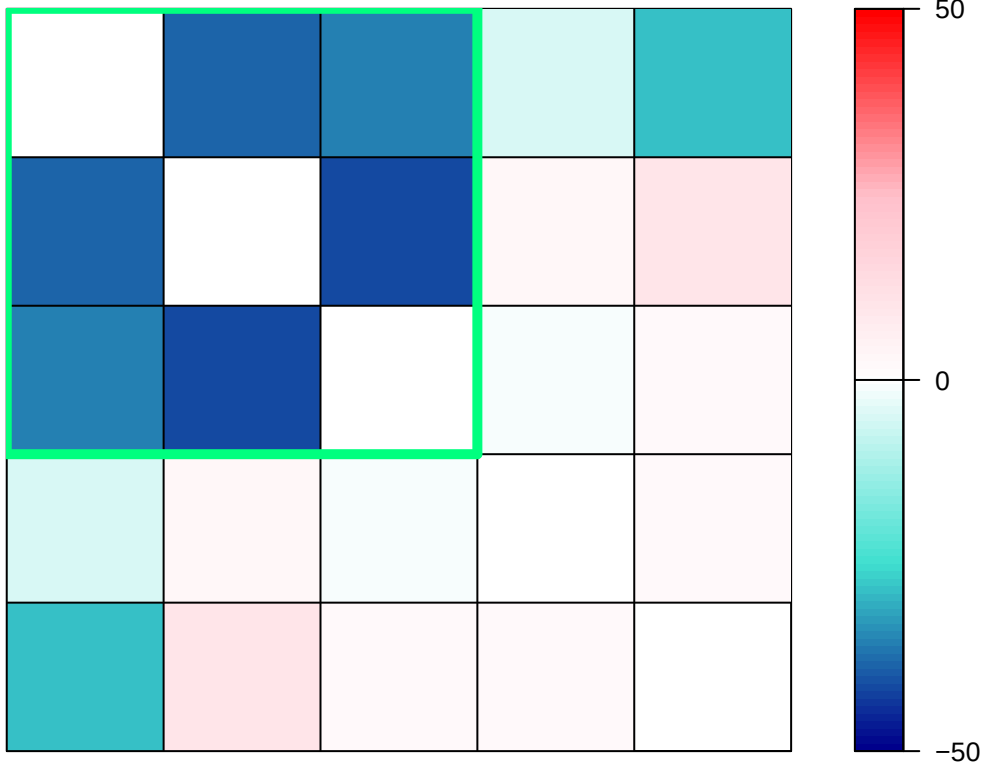
MAE %Diff. (VB2 vs. tICA)
