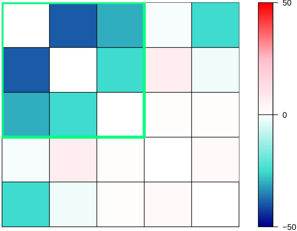
MAE %Diff. (VB1 vs. tICA)
