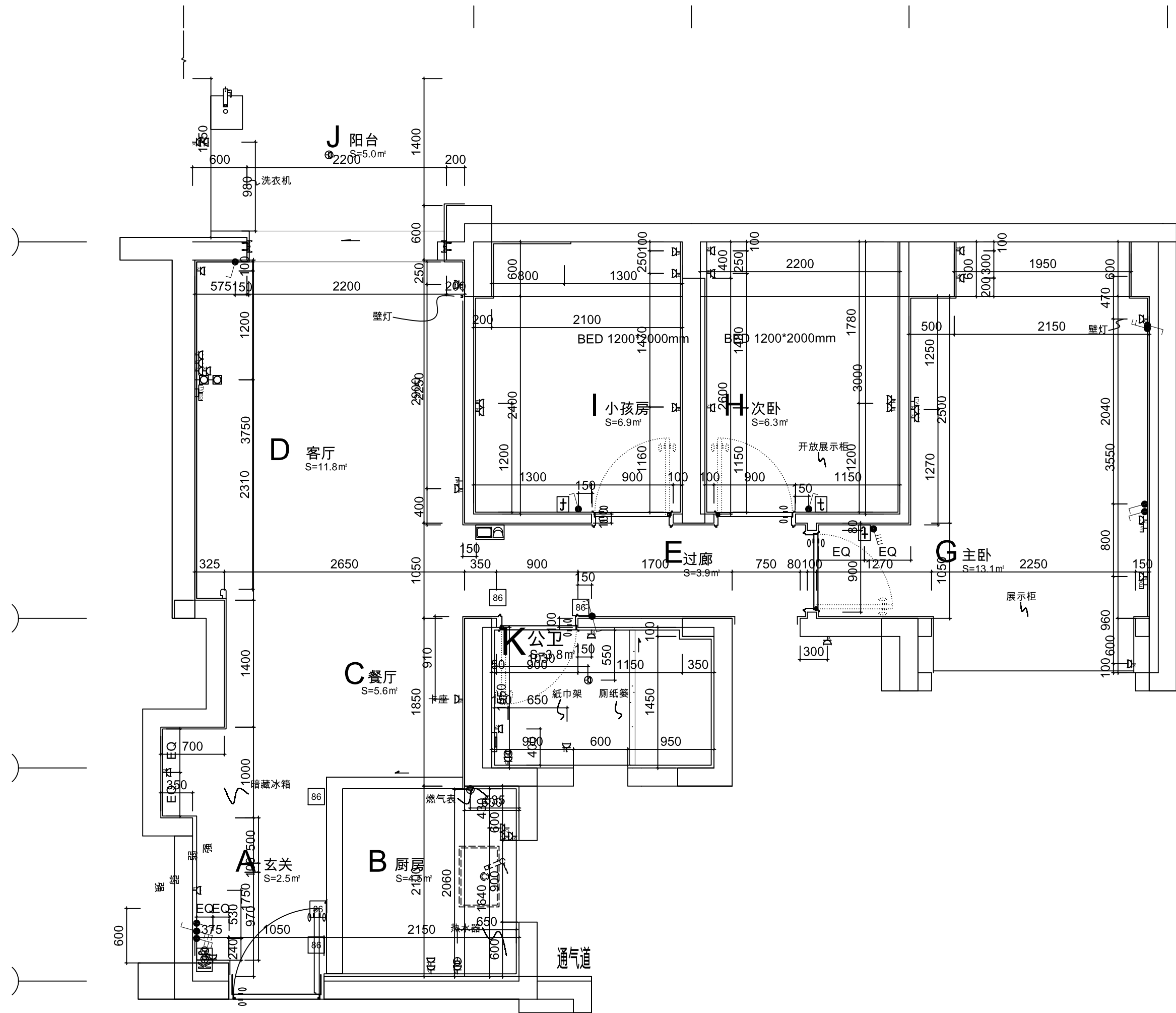
01户型
