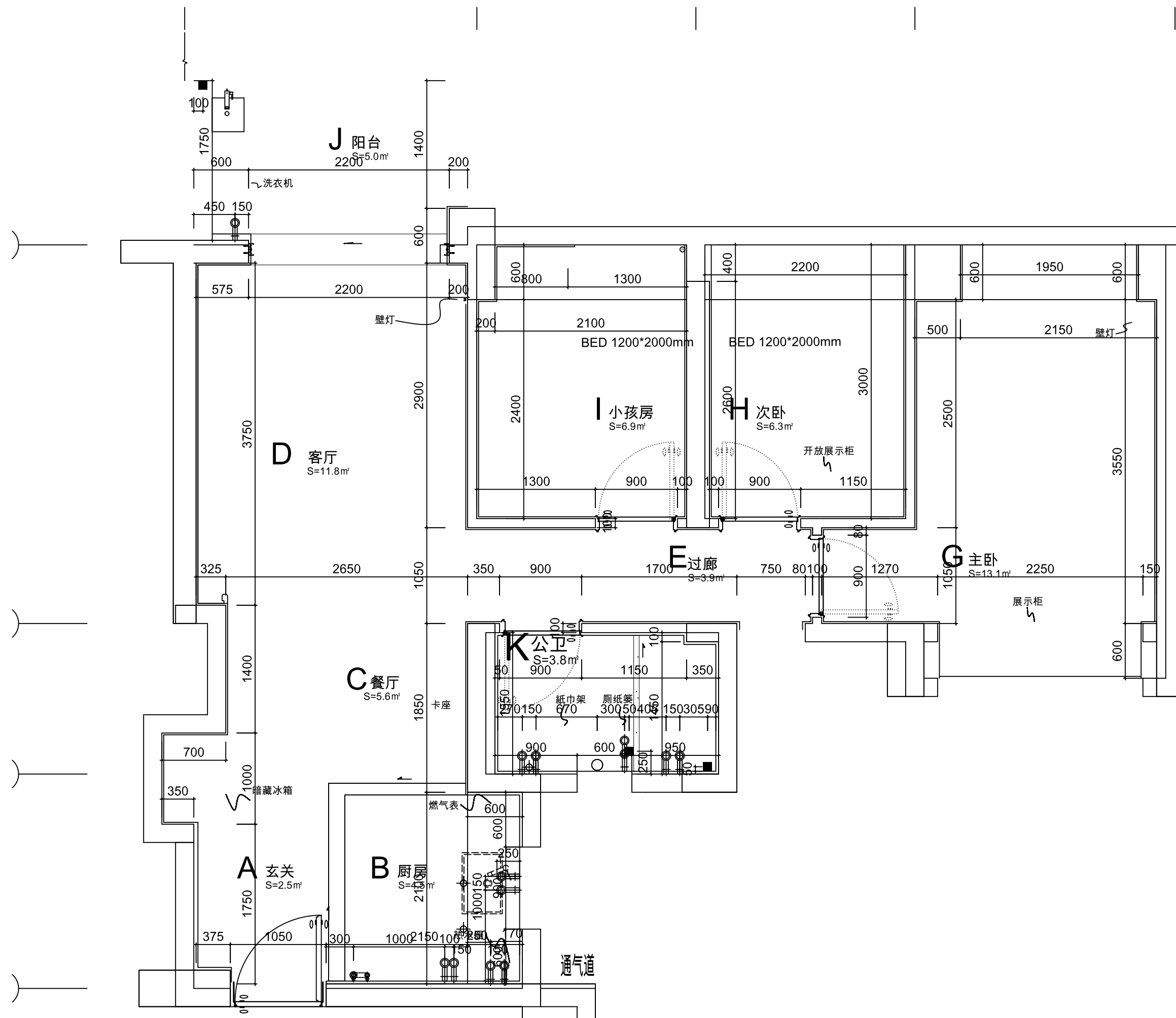
01户型
