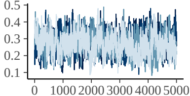
pi_00
