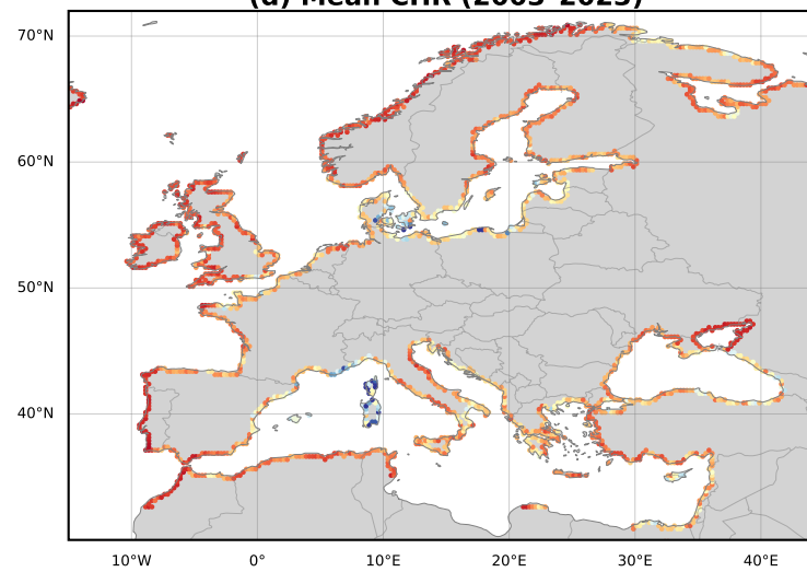
(d) Mean CHR (2003-2023)
