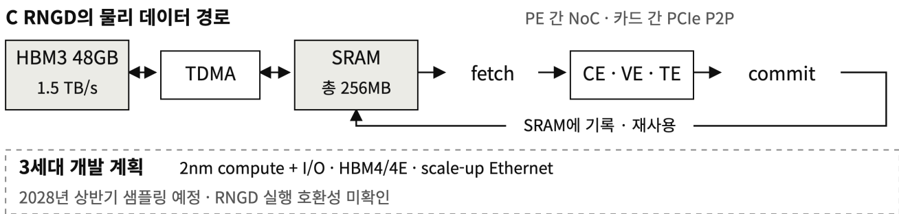
그림 3. 계산 표현·컴파일 산출물·장치 실행을 구분해야 같은 자연 현상에서도 수정할 계층을 찾을 수 있습니다. 공개 자료 재구성이며 3세대는 개발 계획입니다.[6-8]
