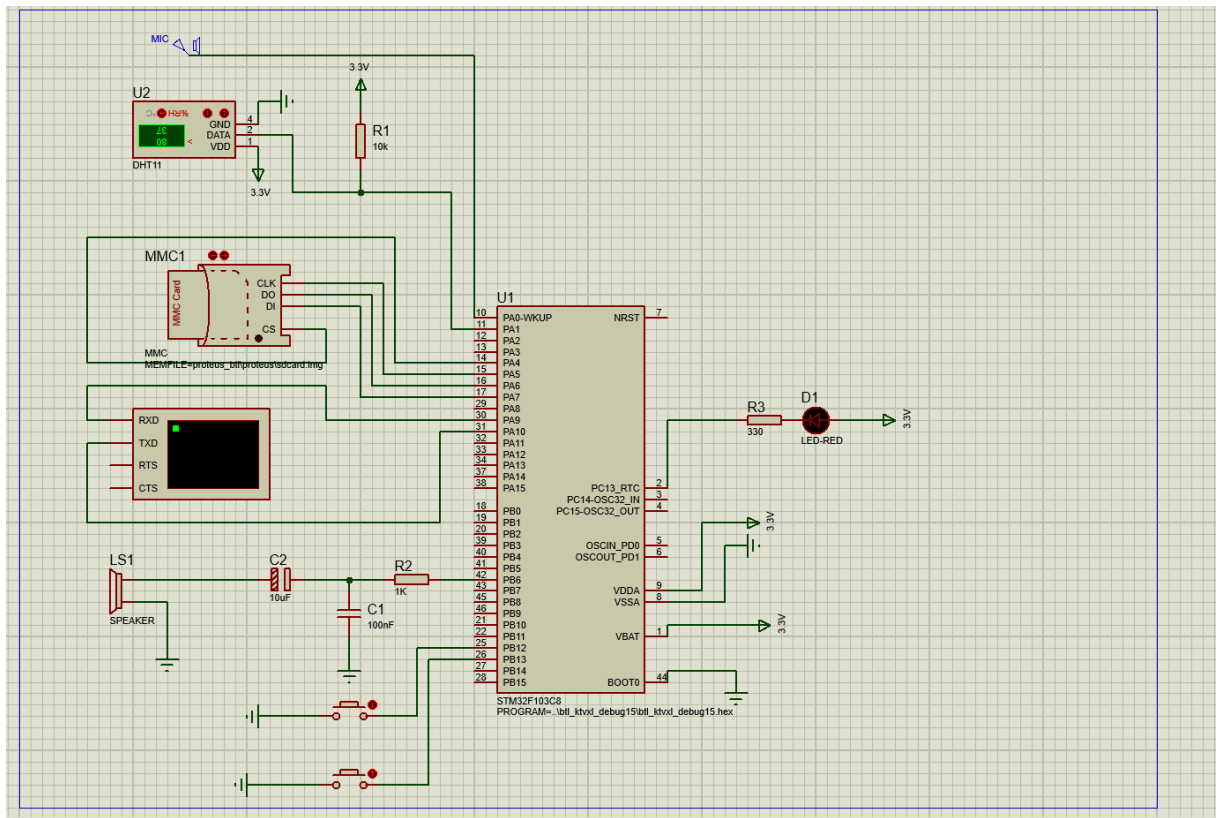
Hình 6. Sơ đồ mạch mô phỏng trên Proteus
