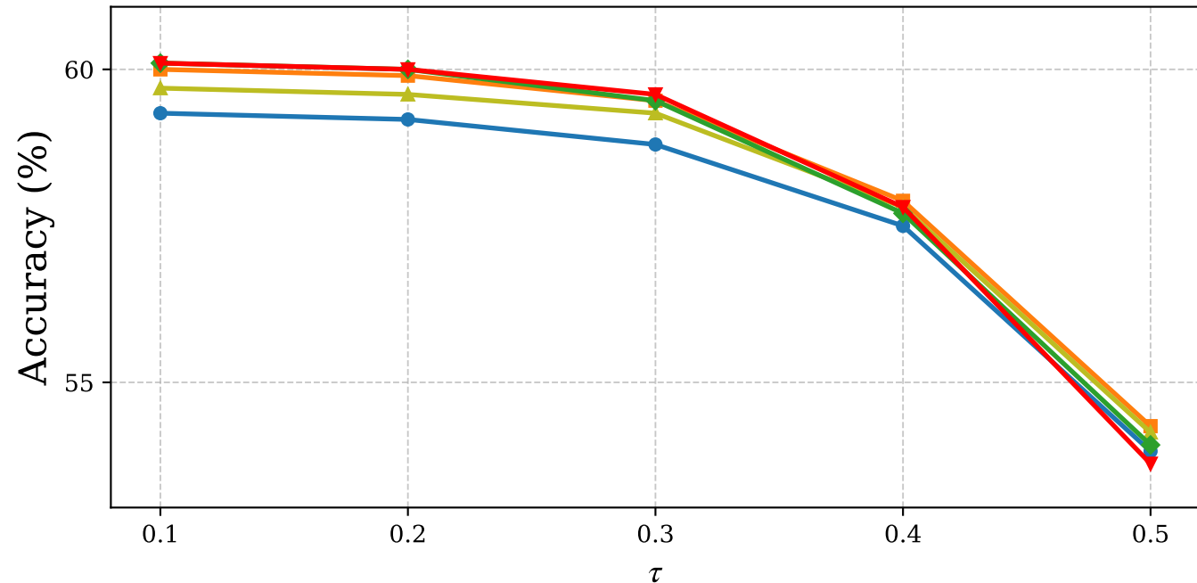
SciQ
