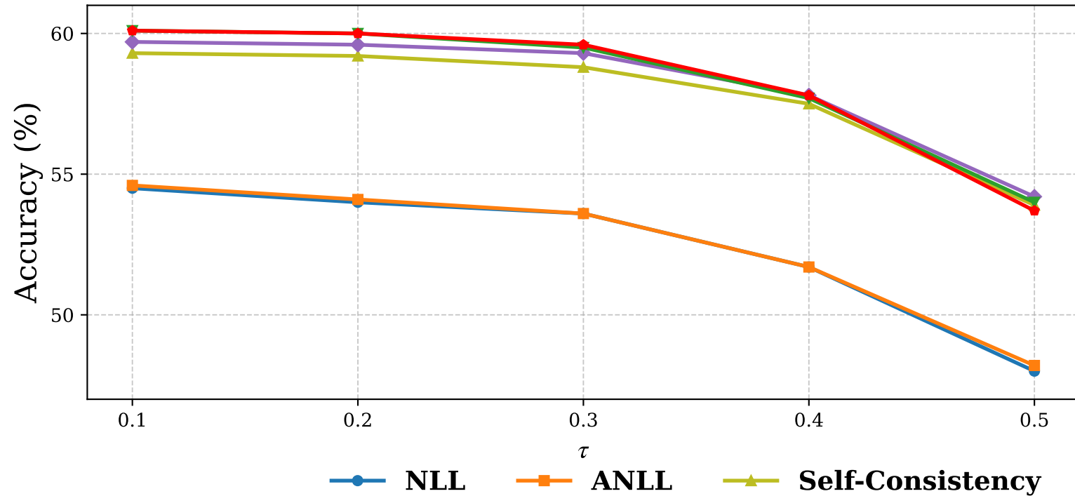
SciQ
