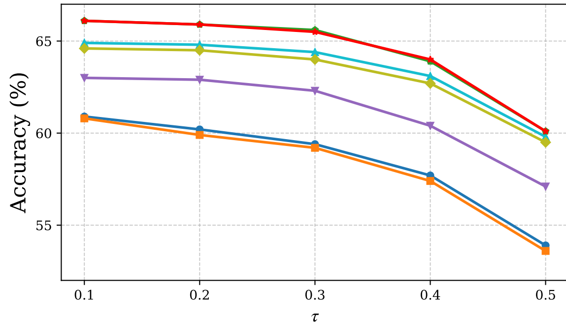
SciQ
