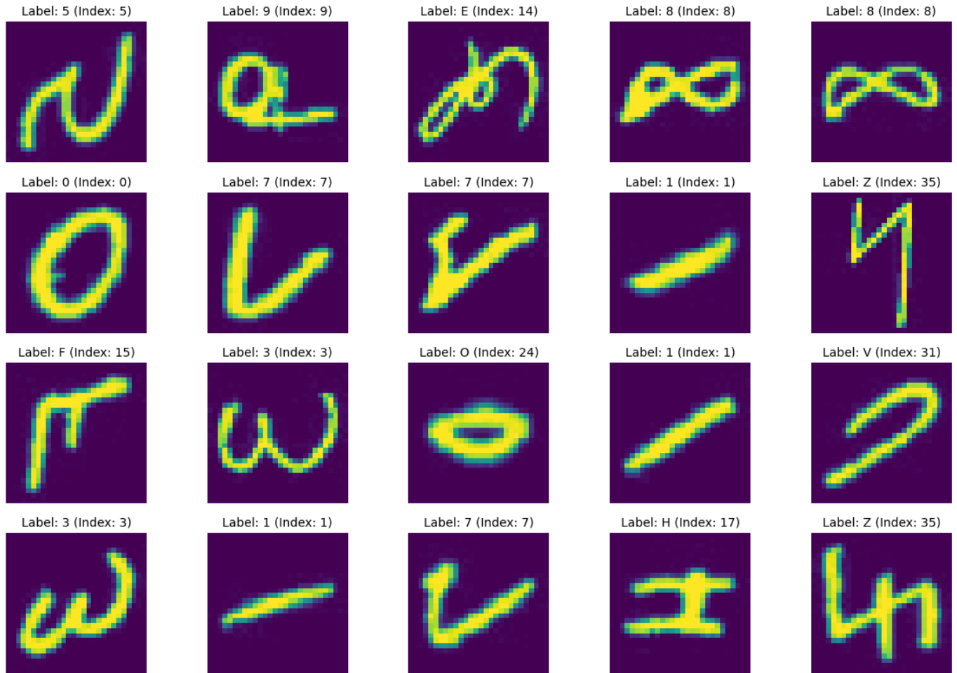
Fig. 1. Dataset Overview
