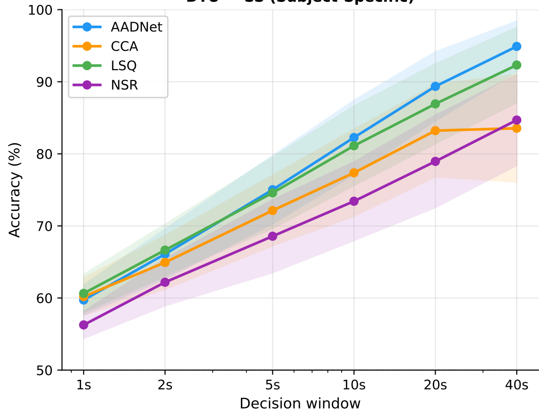
DTU — SS (Subject-Specific)
