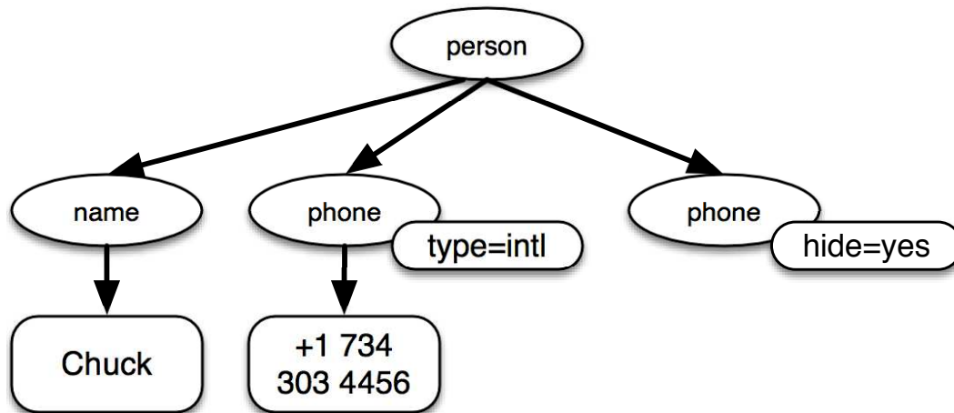
Figure 13.1: Uma representação em árvore de XML
