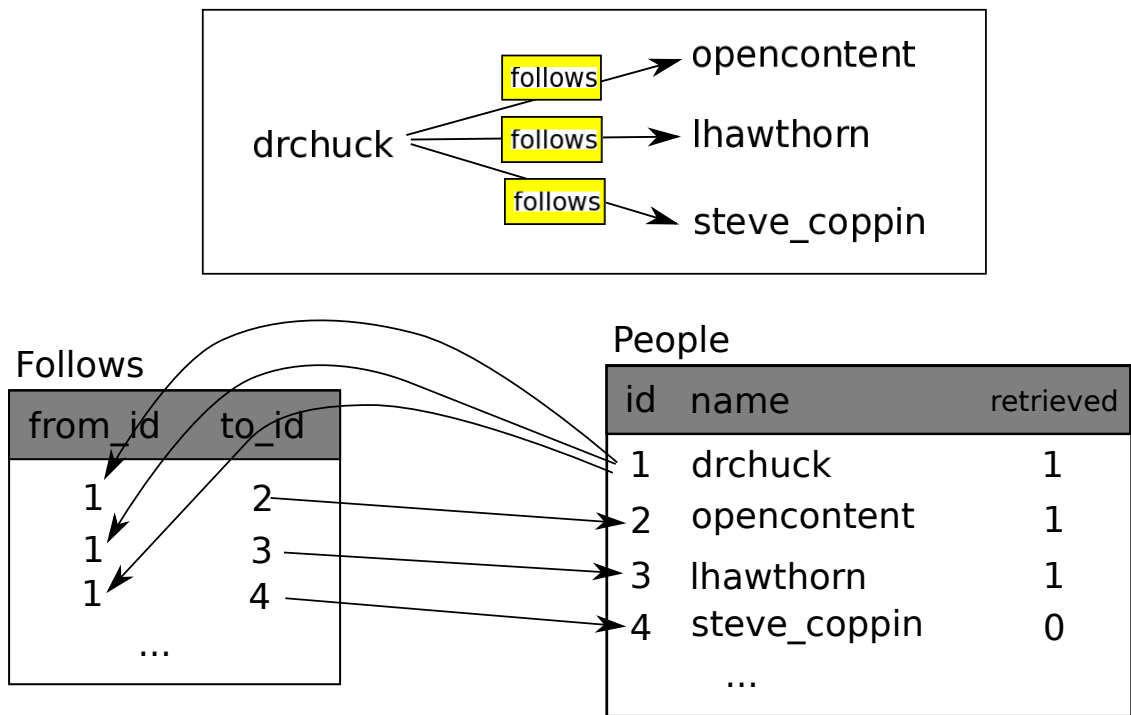
Figure 15.4: Relações Entre Tabelas
