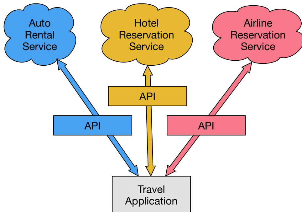
Figure 13.2: Arquitetura Orientada a Serviço
