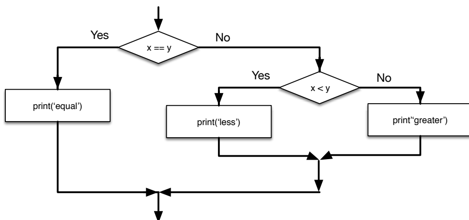
Figure 3.4: Sentenças de if aninhadas
