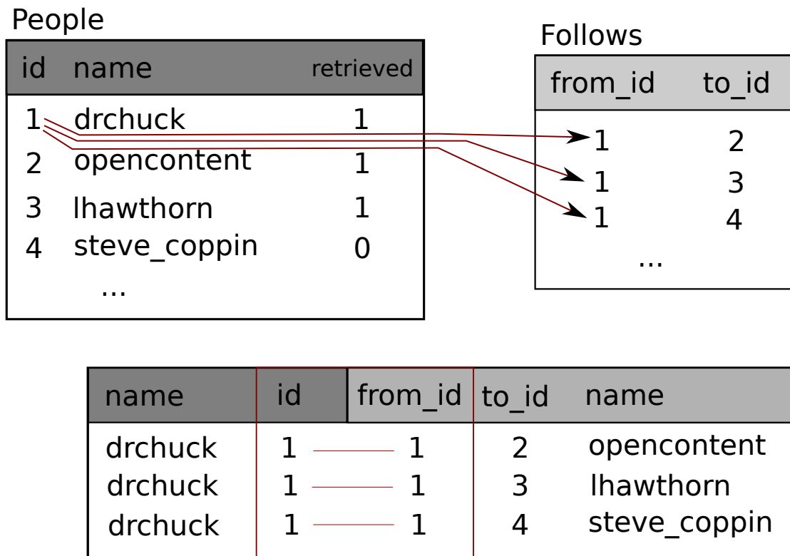
Figure 15.5: Conectando Tabelas Usando JOIN
