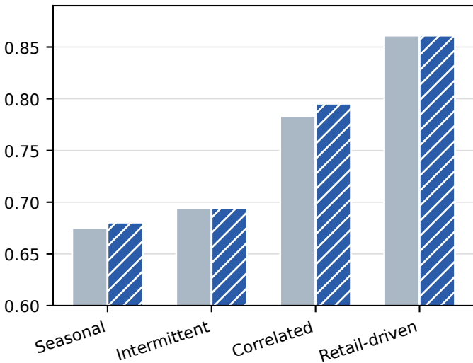
Macro F1
