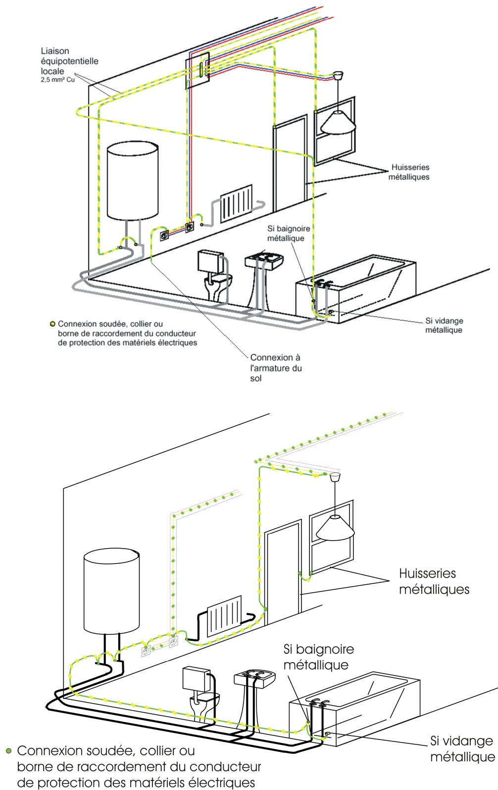
Figures 701E – Exemples de liaison équipotentielle supplémentaire
