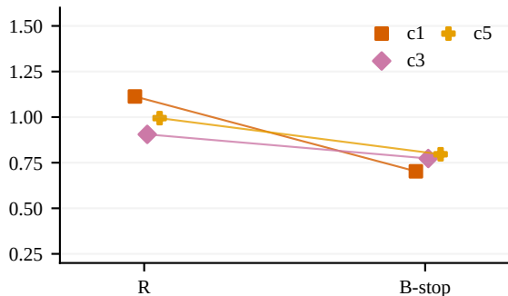
(d) S9, R / B-stop: 3 pairs Unequal lengths; no AUC
